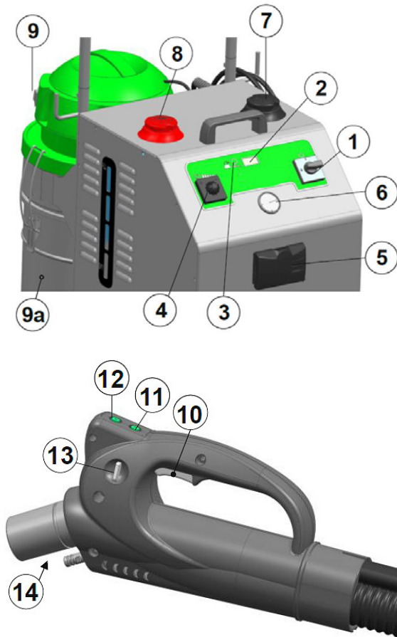
Abb. 3: Gerätebeschreibung SG 58 S
