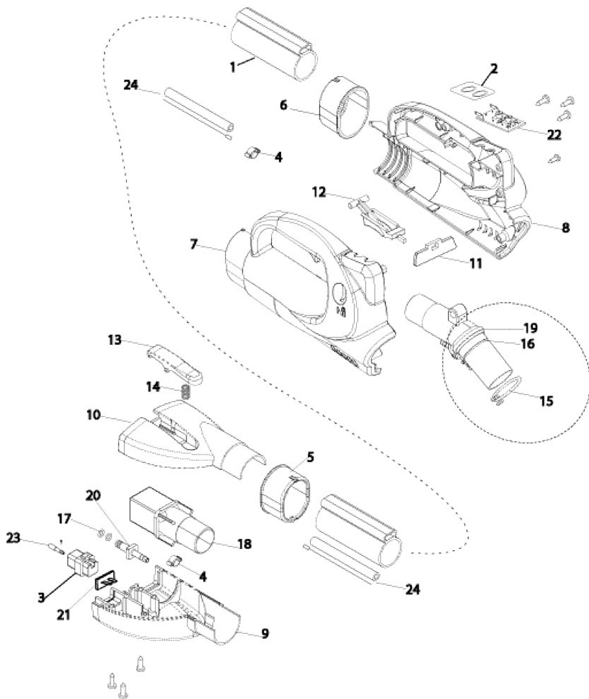
Abb. 19: Ersatzteilzeichnung 3
