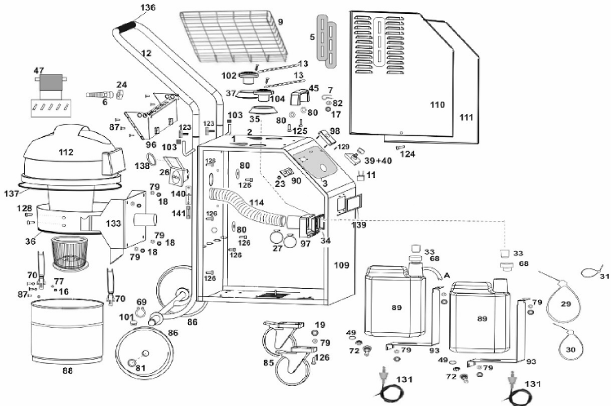
Abb. 17: Ersatzteilzeichnung 1
