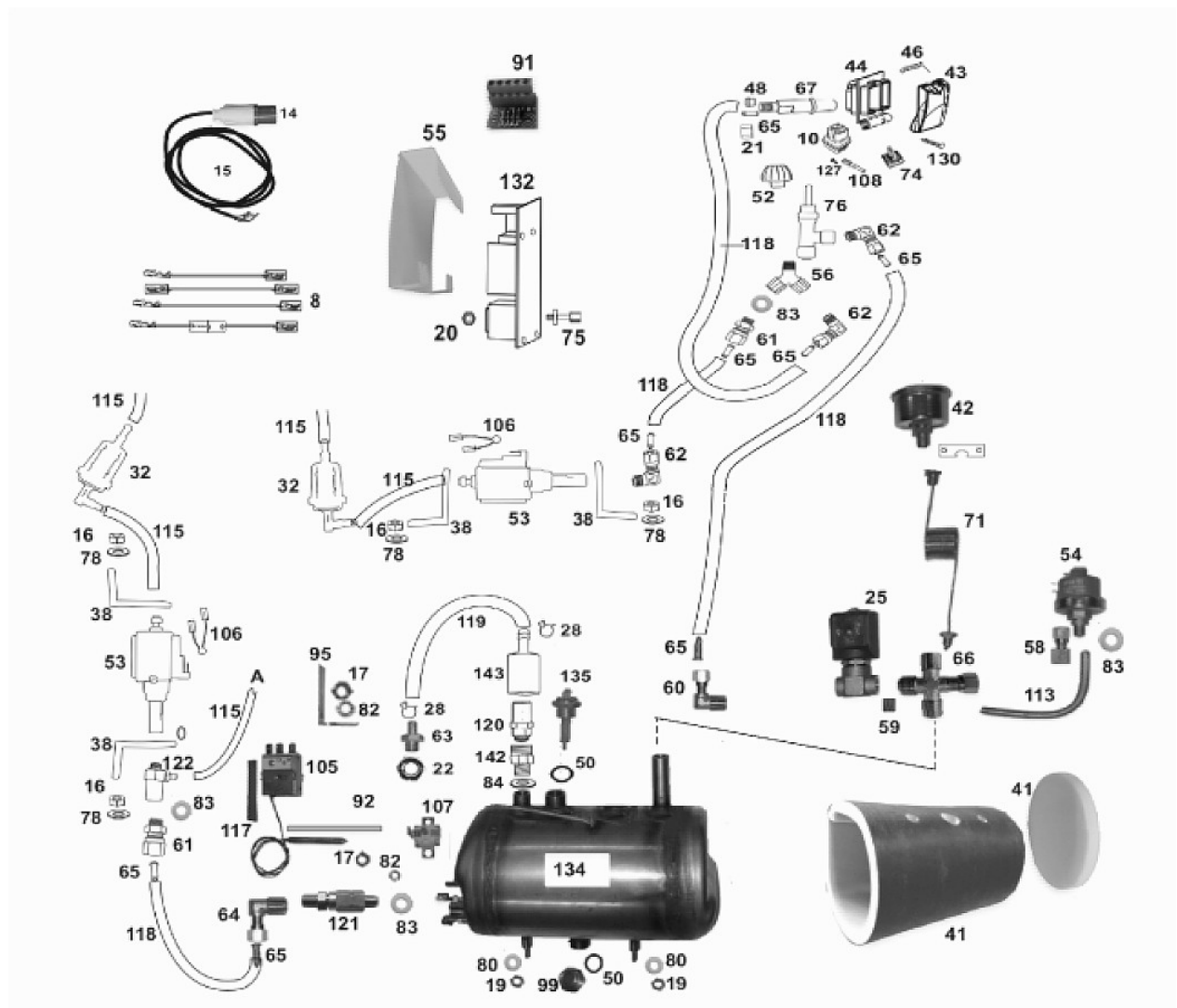
Abb. 18: Ersatzteilzeichnung 2
