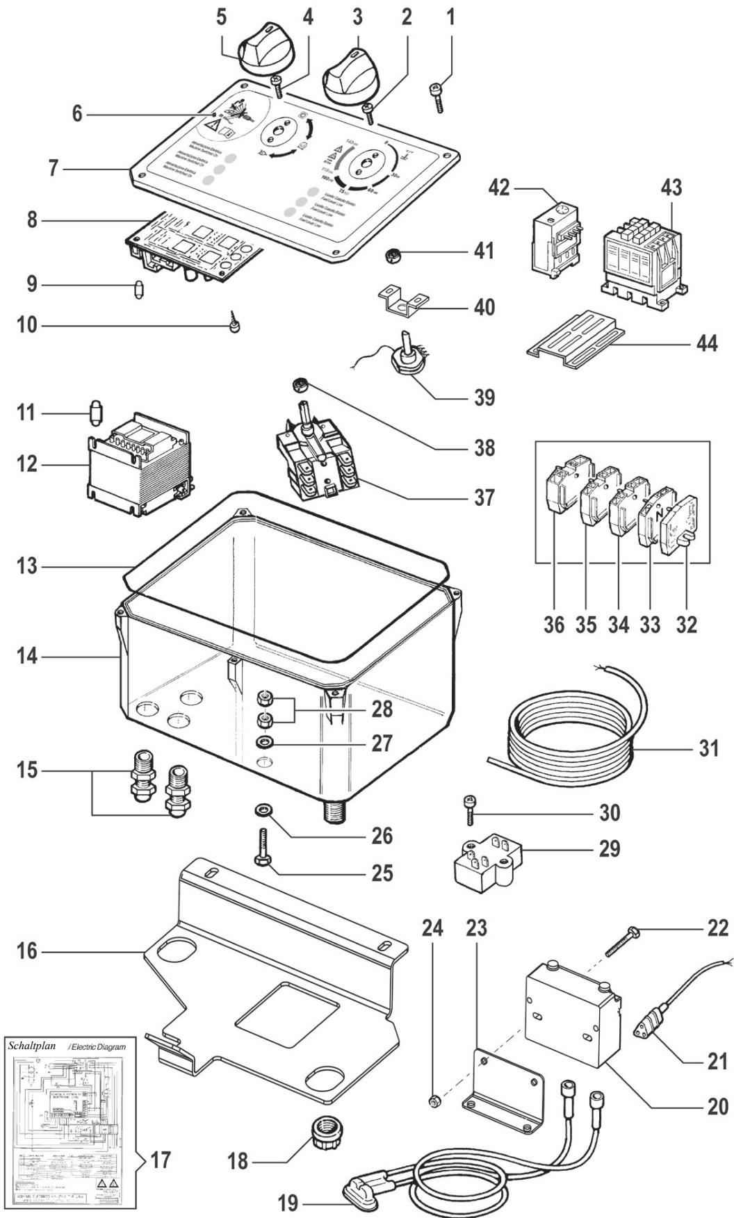
Abb. 14: Ersatzteilzeichnung 6
