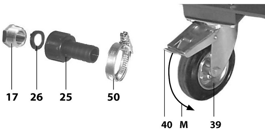
Abb. 6: Beschreibung, Teil 3
