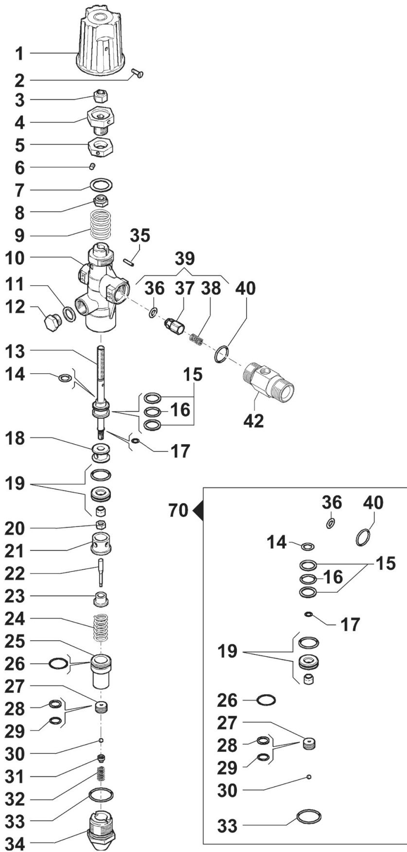
Abb. 12: Ersatzteilzeichnung 4
