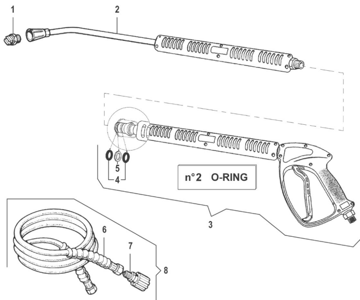
Abb. 16: Ersatzteilzeichnung 8
