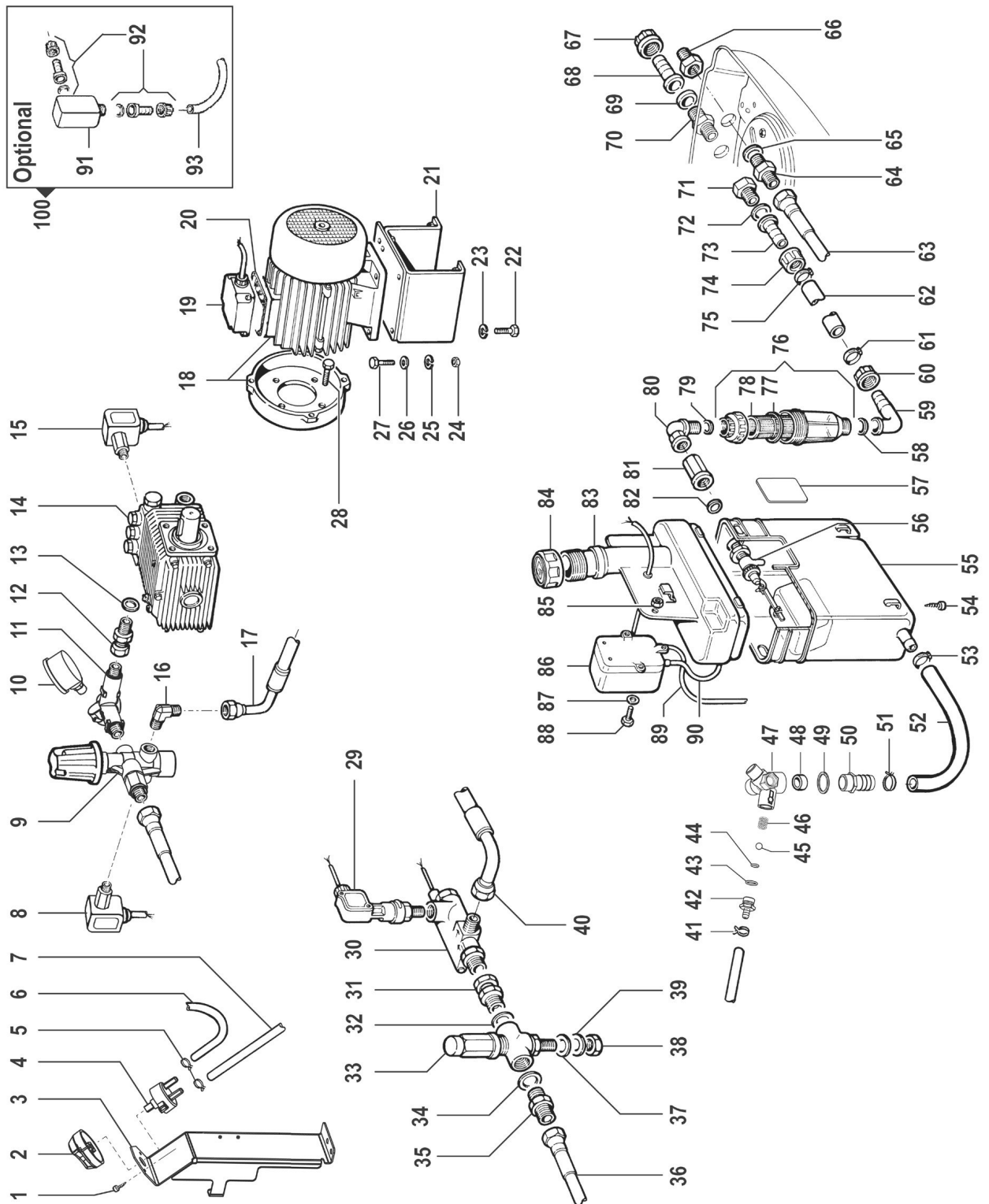
Abb. 13: Ersatzteilzeichnung 5
