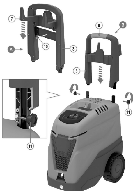
Abb. 4: Gerätebeschreibung Teil 2
