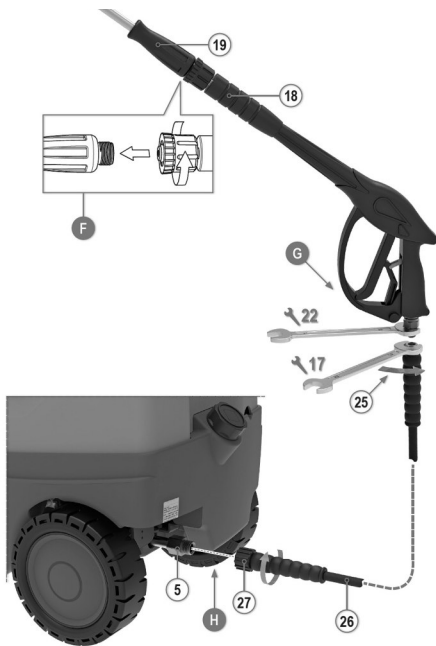
Abb. 9: Montage des Zubehörs Teil 1
