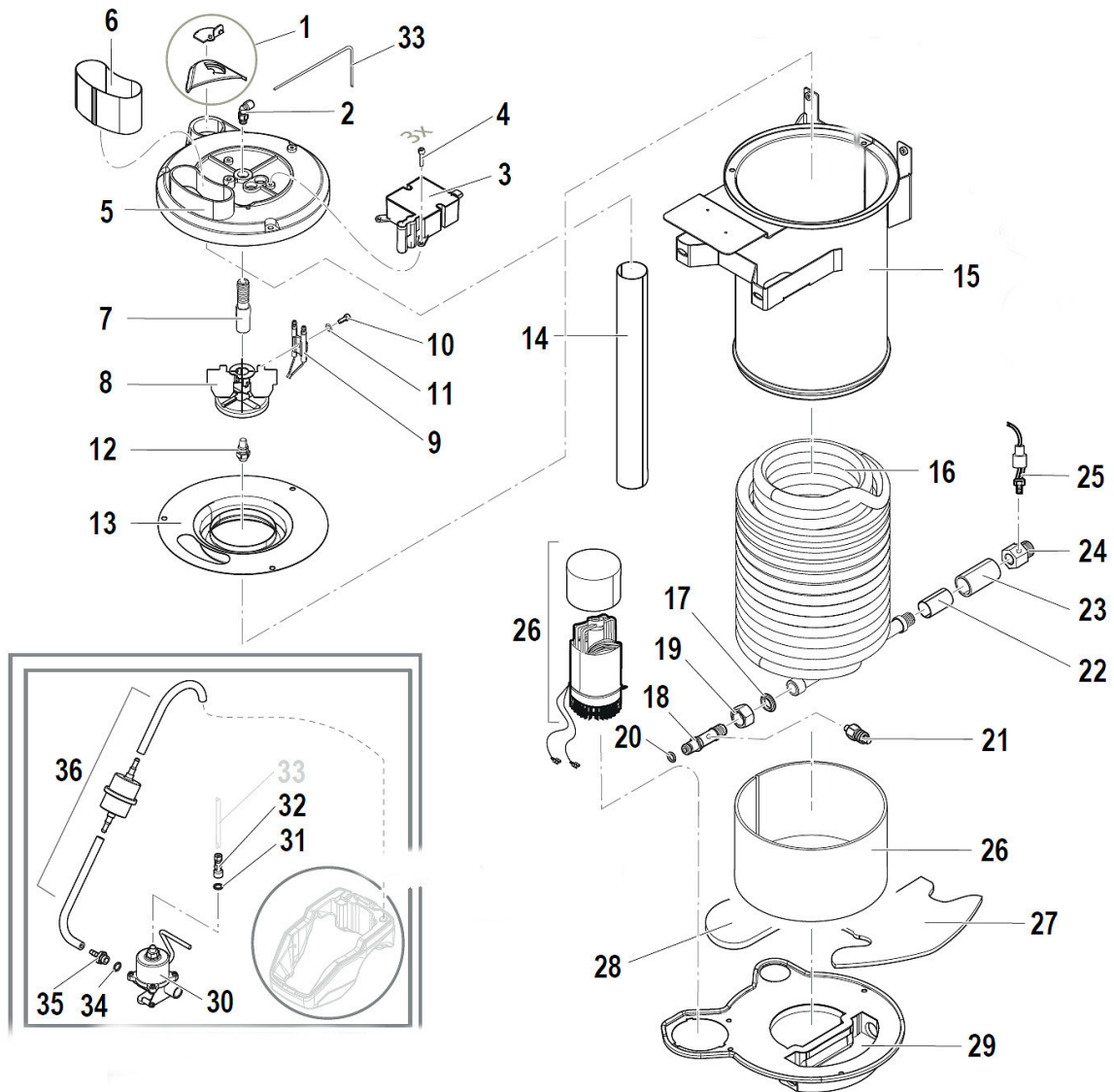
Abb. 20: Ersatzteilzeichnung 5
