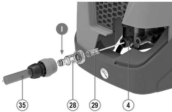
Abb. 6: Gerätebeschreibung Teil 4
