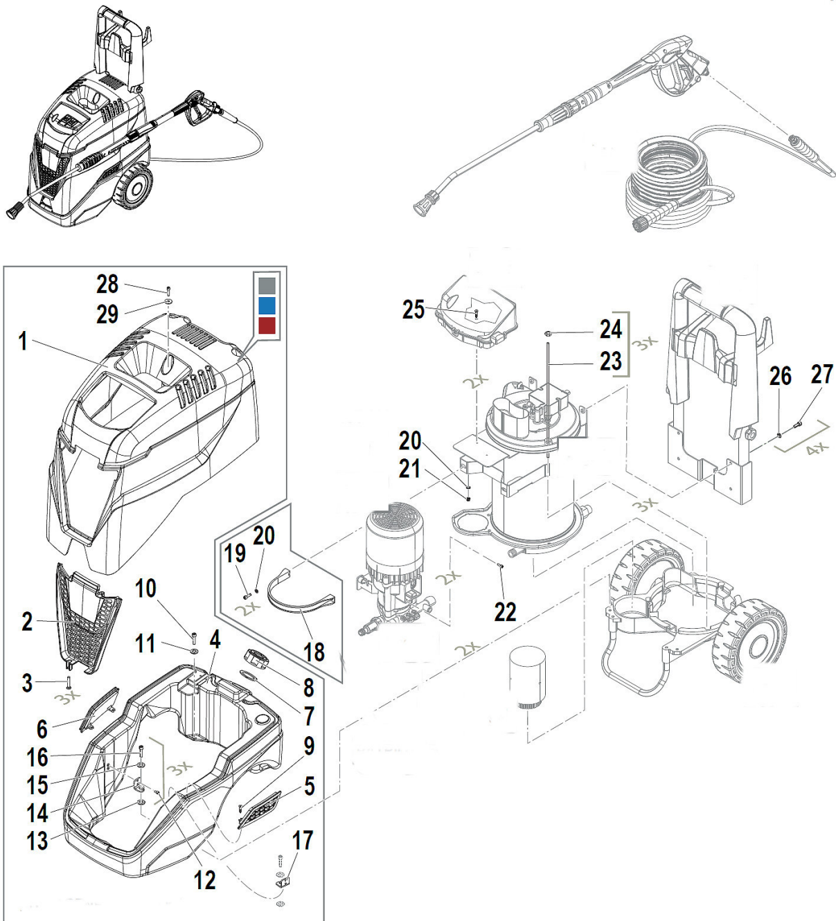
Abb. 16: Ersatzteilzeichnung 1
