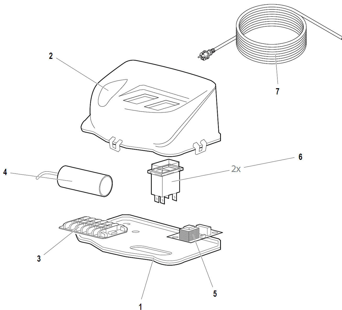
Abb. 18: Ersatzteilzeichnung 3
