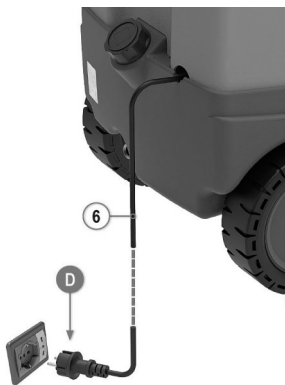
Abb. 13: Vorbereitung für den Betrieb Teil 3
