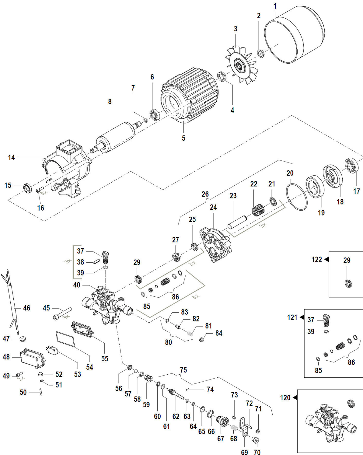
Abb. 21: Ersatzteilzeichnung 6
