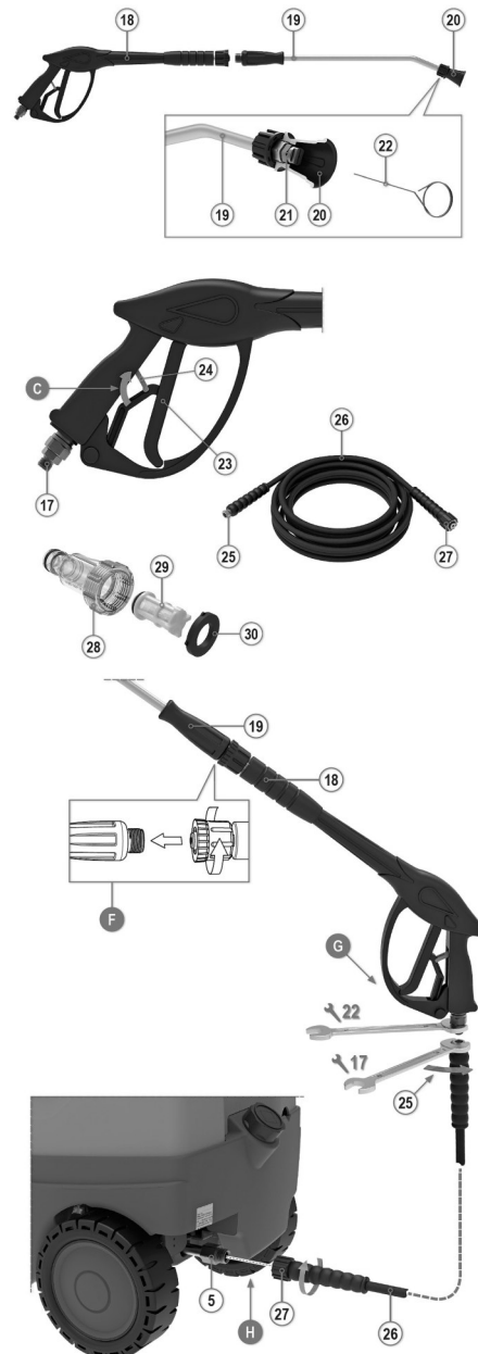
Abb. 5: Gerätebeschreibung Teil 3
