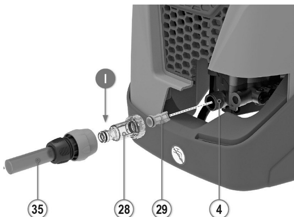
Abb. 10: Montage des Zubehörs Teil 2
