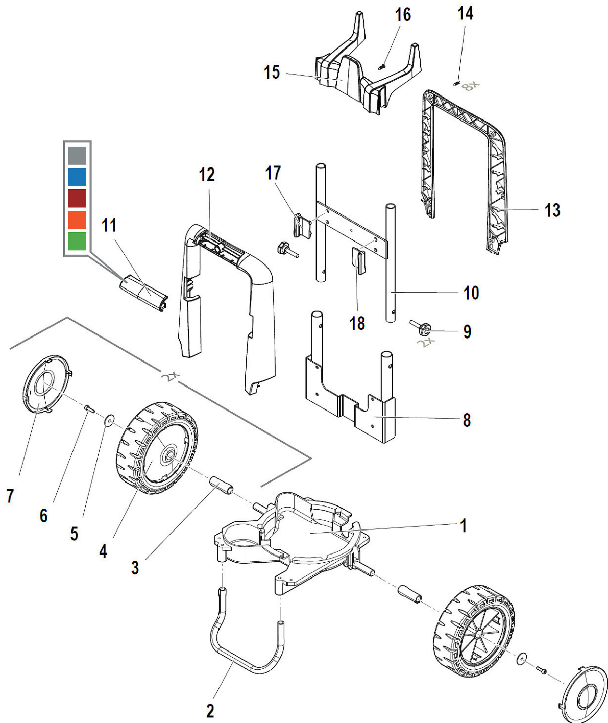
Abb. 17: Ersatzteilzeichnung 2
