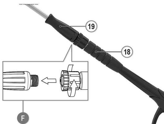
Abb. 14: Vorbereitung für den Betrieb Teil 4
