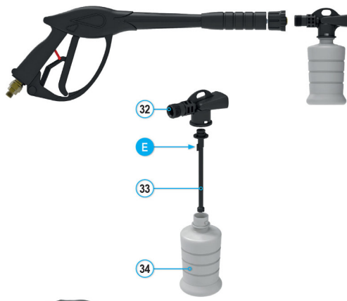
Abb. 15: Betrieb mit Reinigungsmittel
