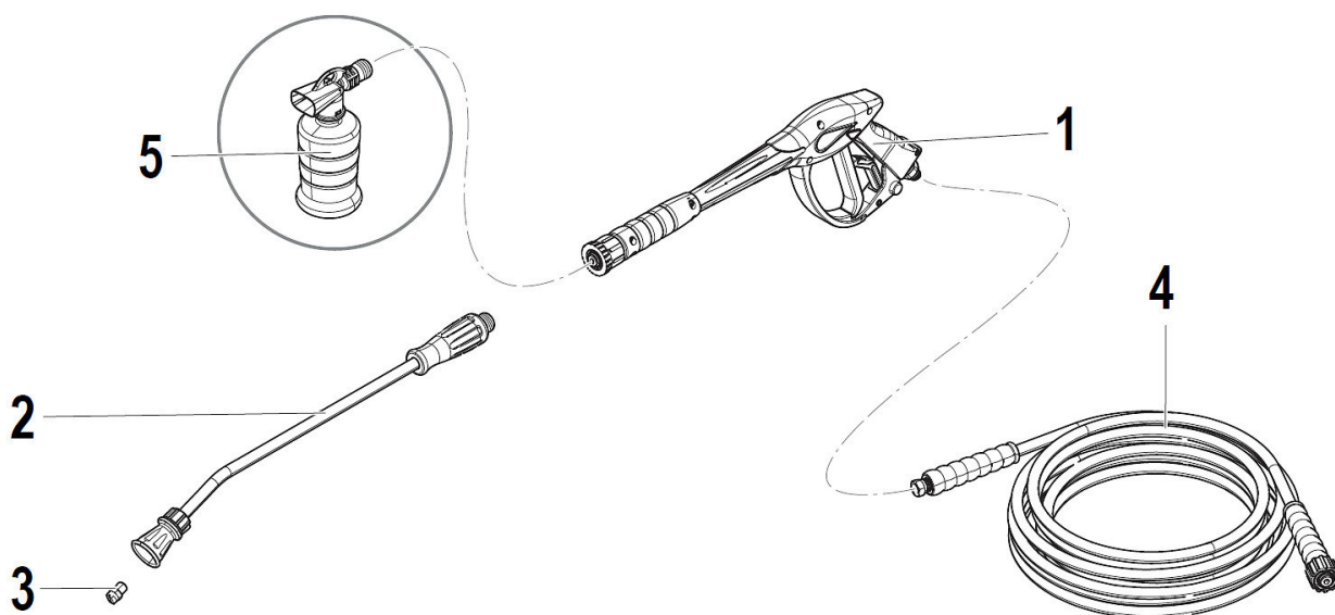
Abb. 19: Ersatzteilzeichnung 4
