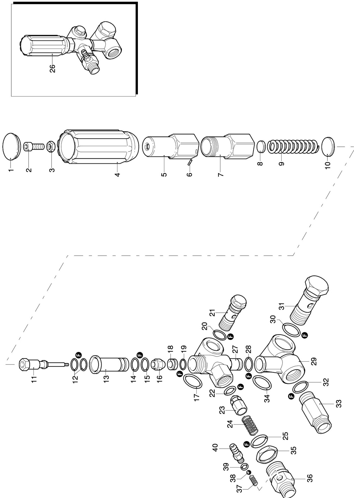
Abb. 14: Ersatzteilzeichnung 3
