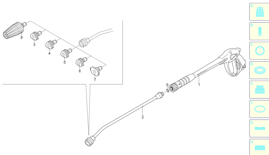
Abb. 15: Ersatzteilzeichnungen 4 und 5
