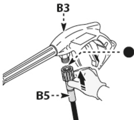
Abb. 7: Montage
