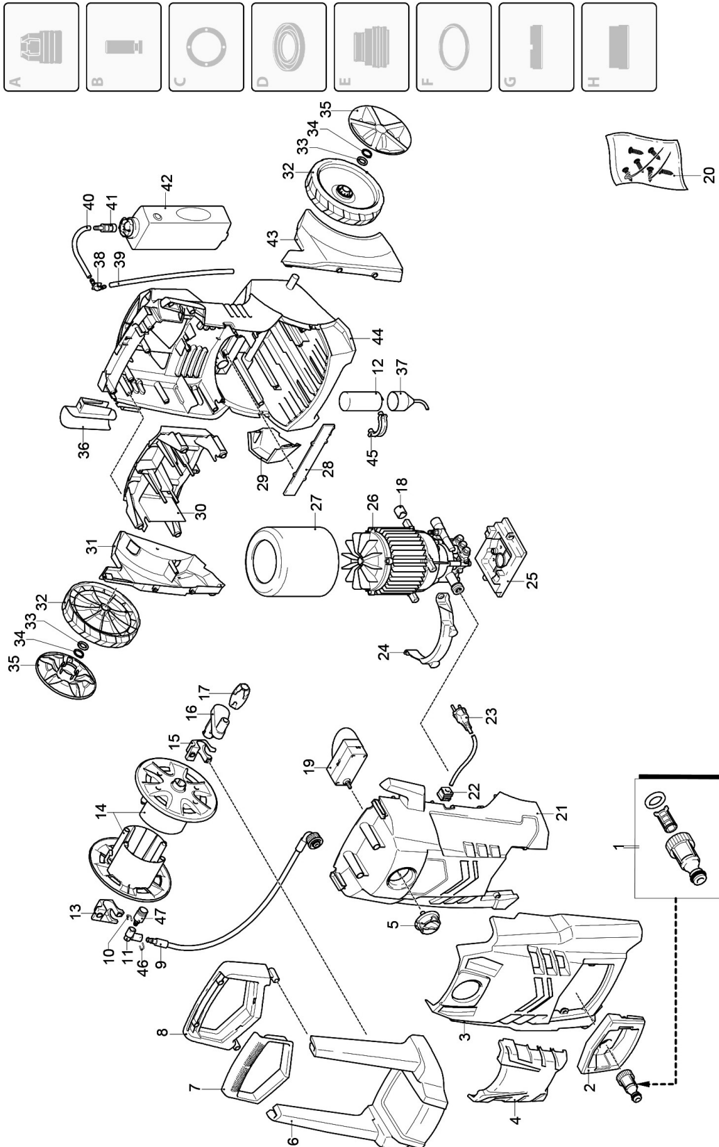
Abb. 14: Ersatzteilzeichnung 1
