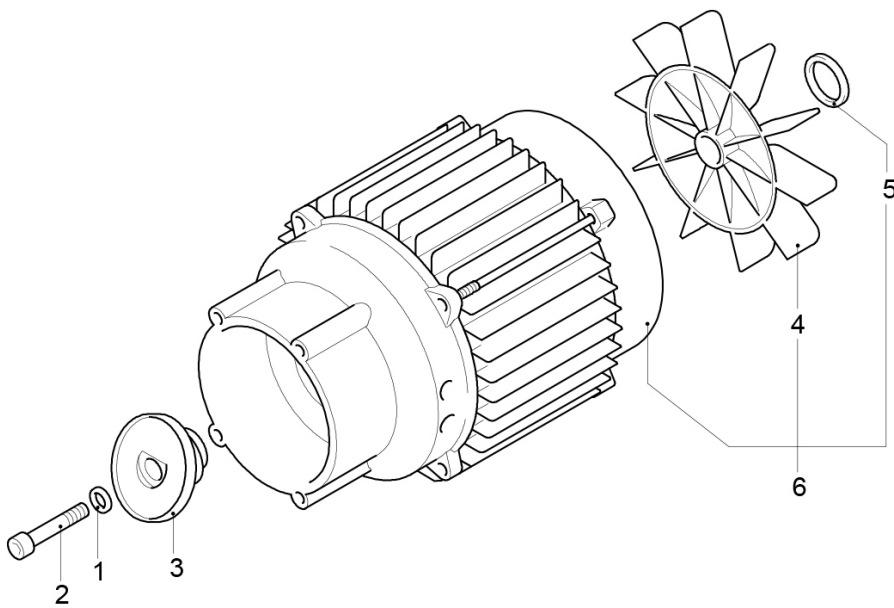
Abb. 16: Ersatzteilzeichnung 3
