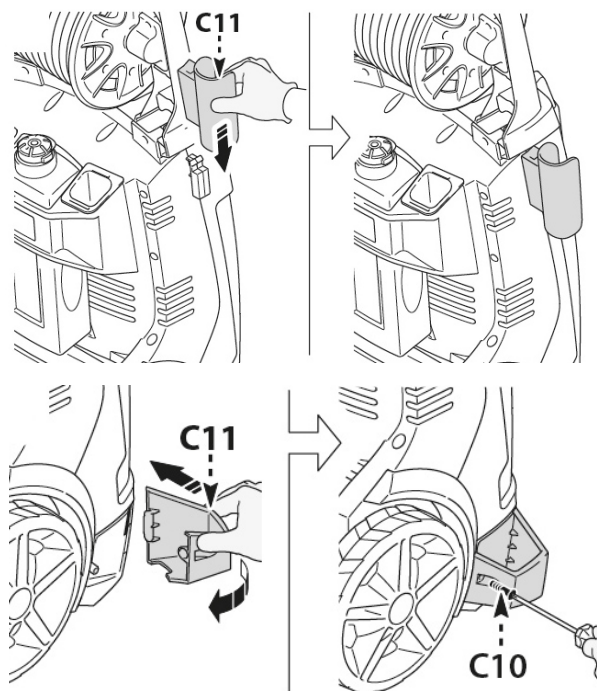
Abb. 6: Montage
