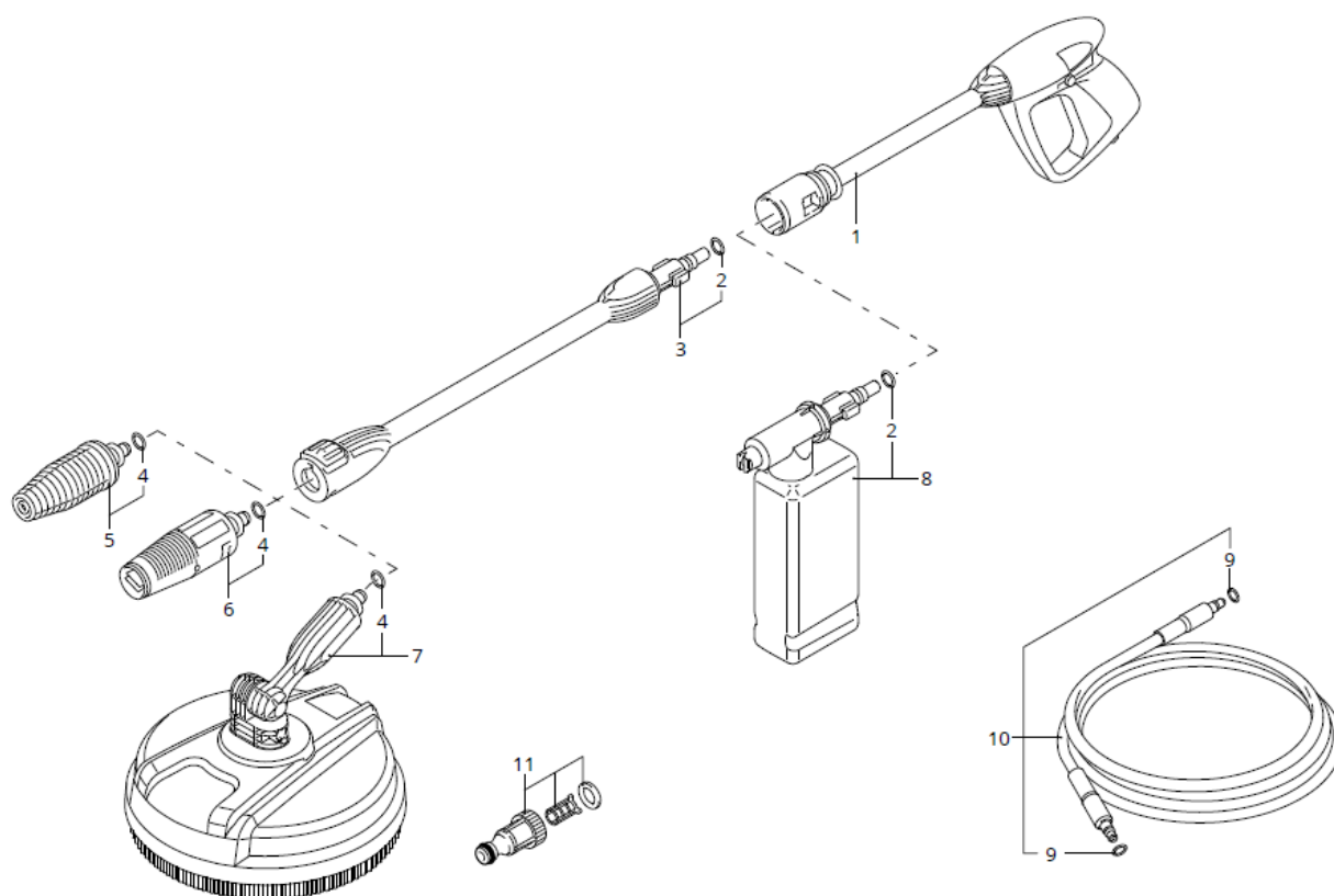
Abb.9-3: Ersatzteilzeichnung 3
