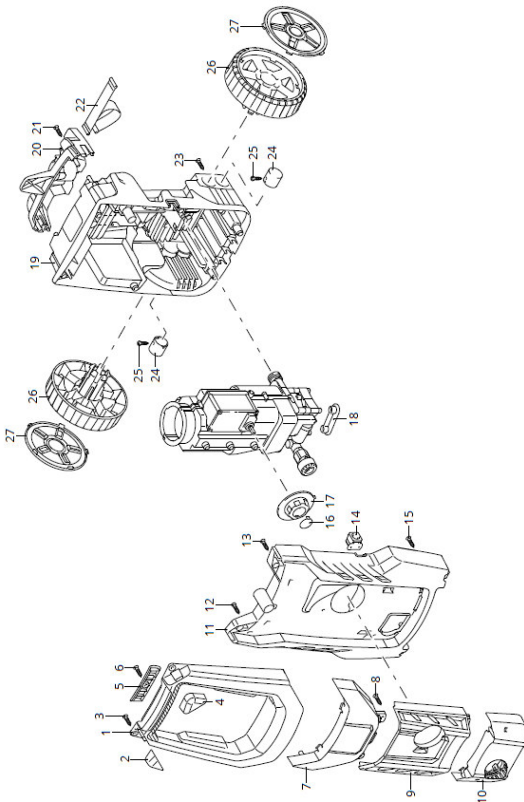
Abb.9-1: Ersatzteilzeichnungen 1
