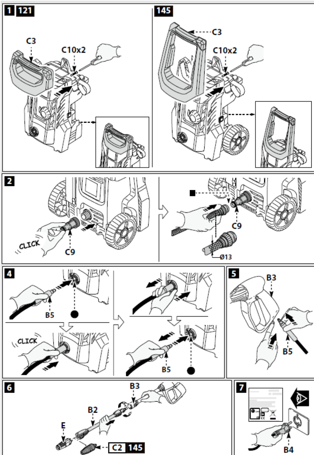
Abb. 5-1: Visuelle Montageanleitung
