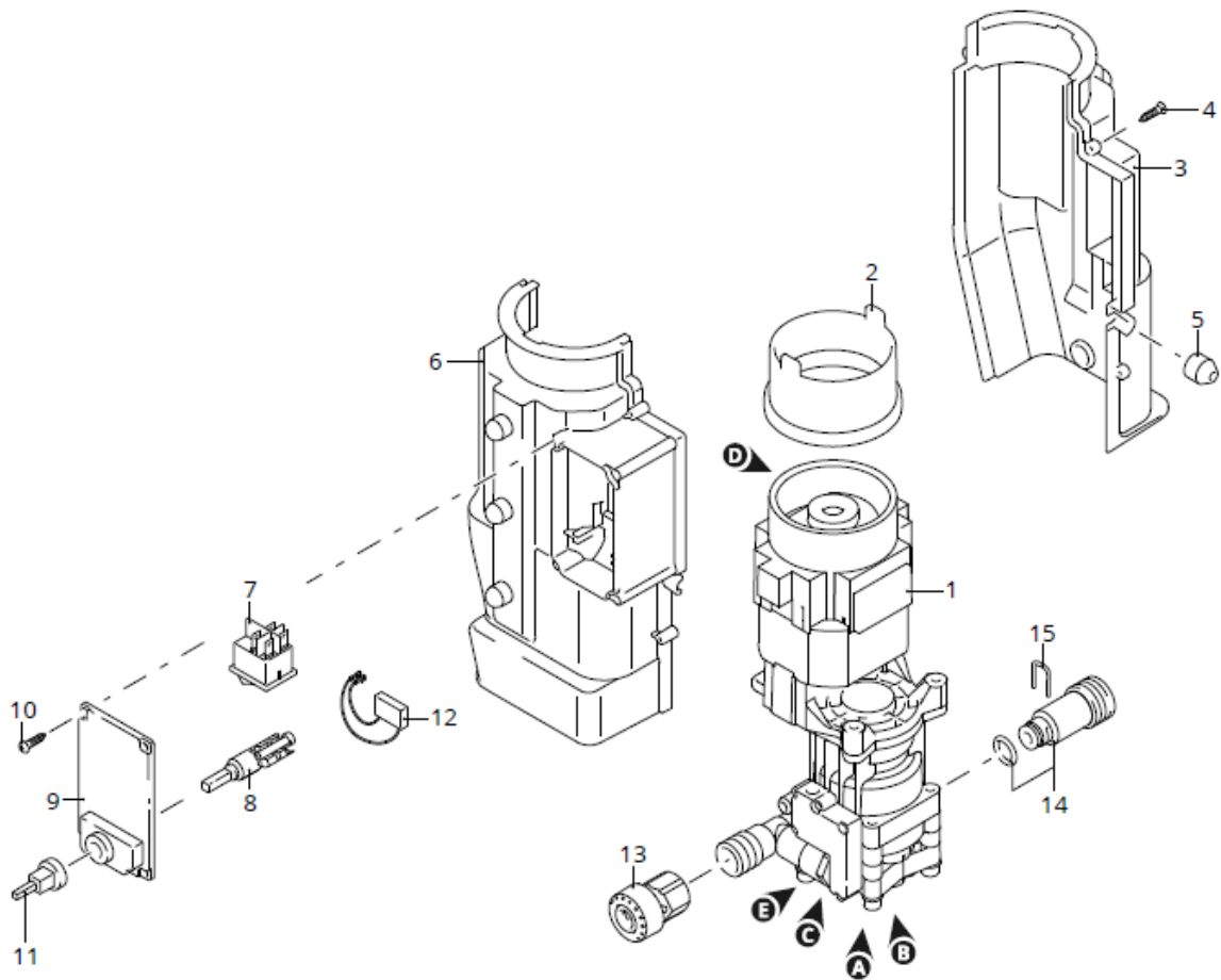
Abb. 9-2: Ersatzteilzeichnungen 2
