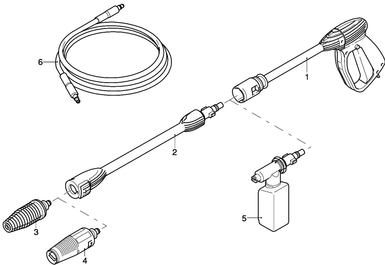
Abb. 12: Ersatzteilzeichnung 2
