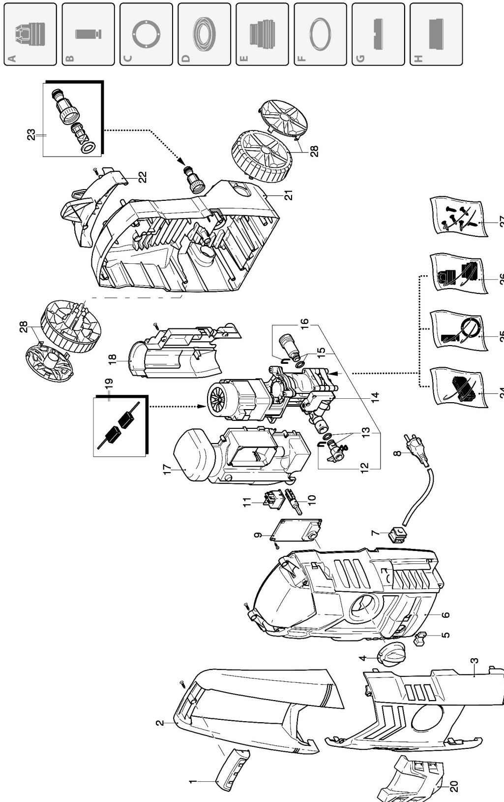
Abb. 11: Ersatzteilzeichnung 1
