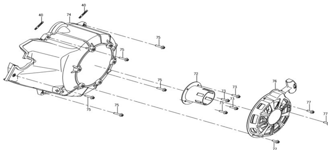
Abb. 10-35: Ersatzteilzeichnung 7
