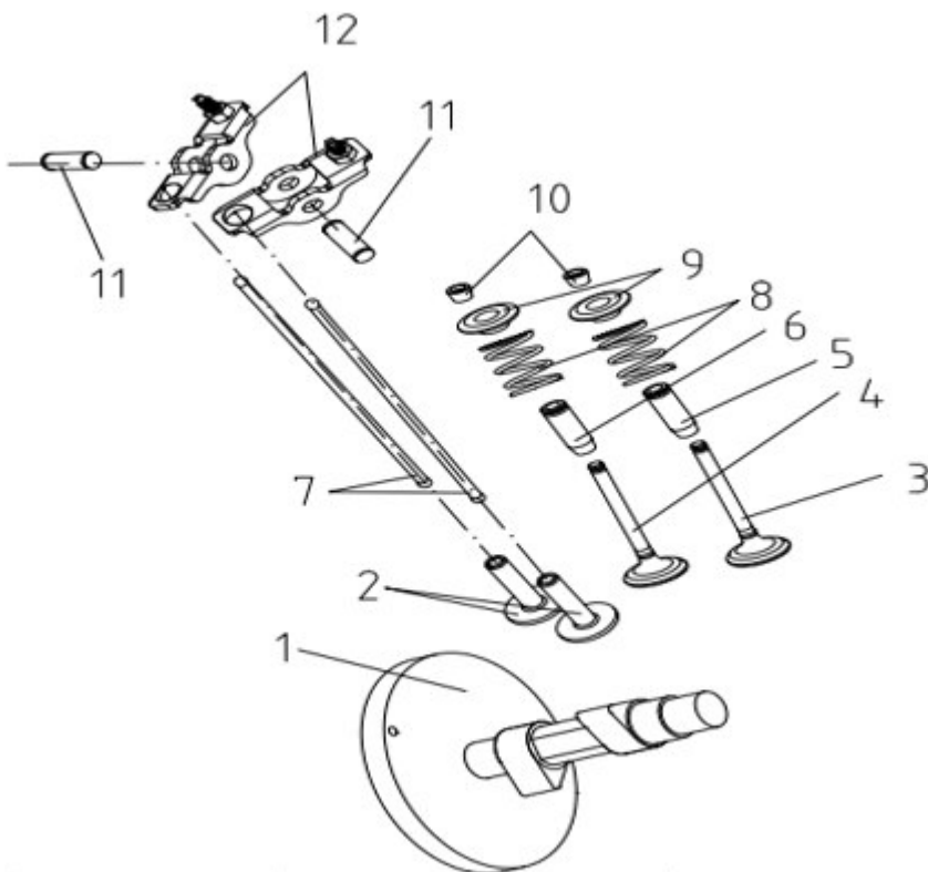
Abb. 10-6: Ersatzteilzeichnung 5
