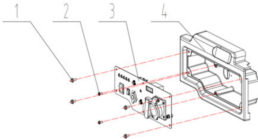
Abb. 10-27: Ersatzteilzeichnung 8
