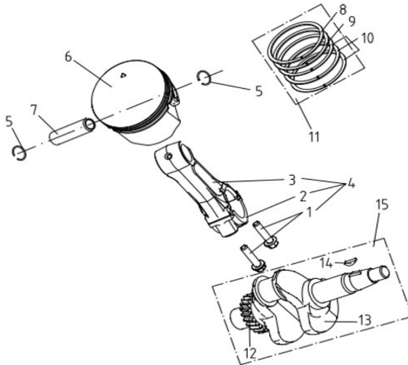
Abb. 10-5: Ersatzteilzeichnung 4
