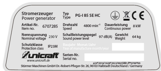
Abb.2-1: Typenschild PG-I 85 SE HC
