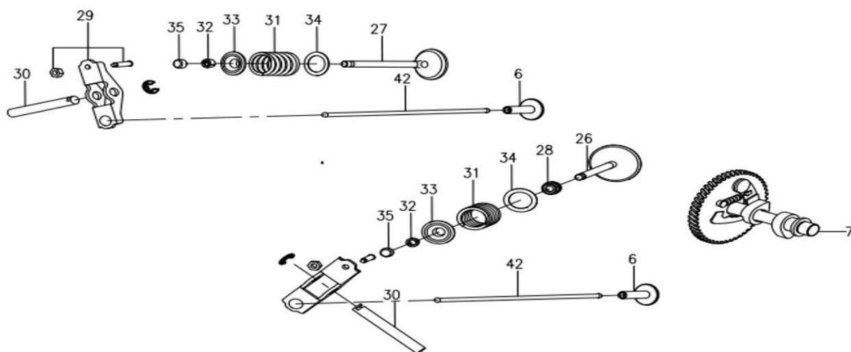
Abb. 10-34: Ersatzteilzeichnung 6
