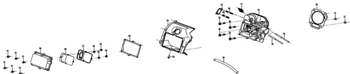
Abb. 10-30: Ersatzteilzeichnung 2
