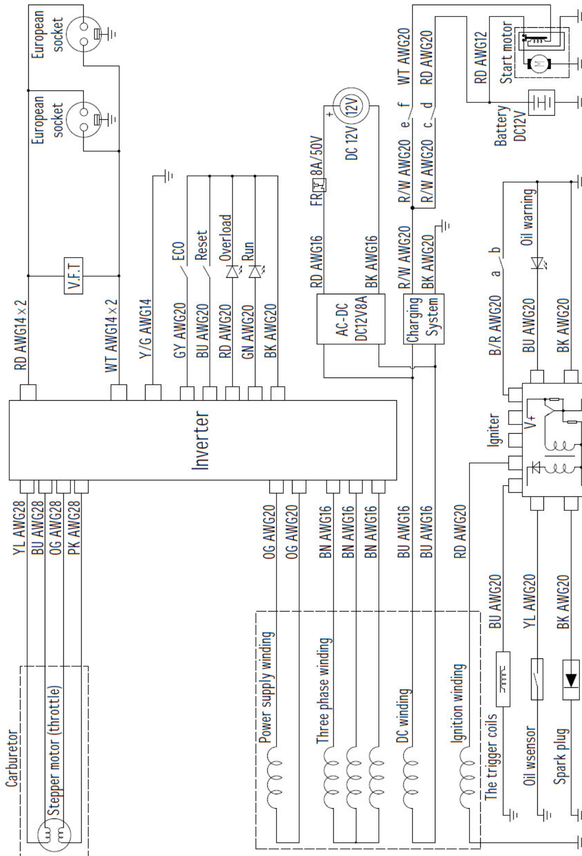
Abb. 11-3: Schaltplan PG-I 41 SE
