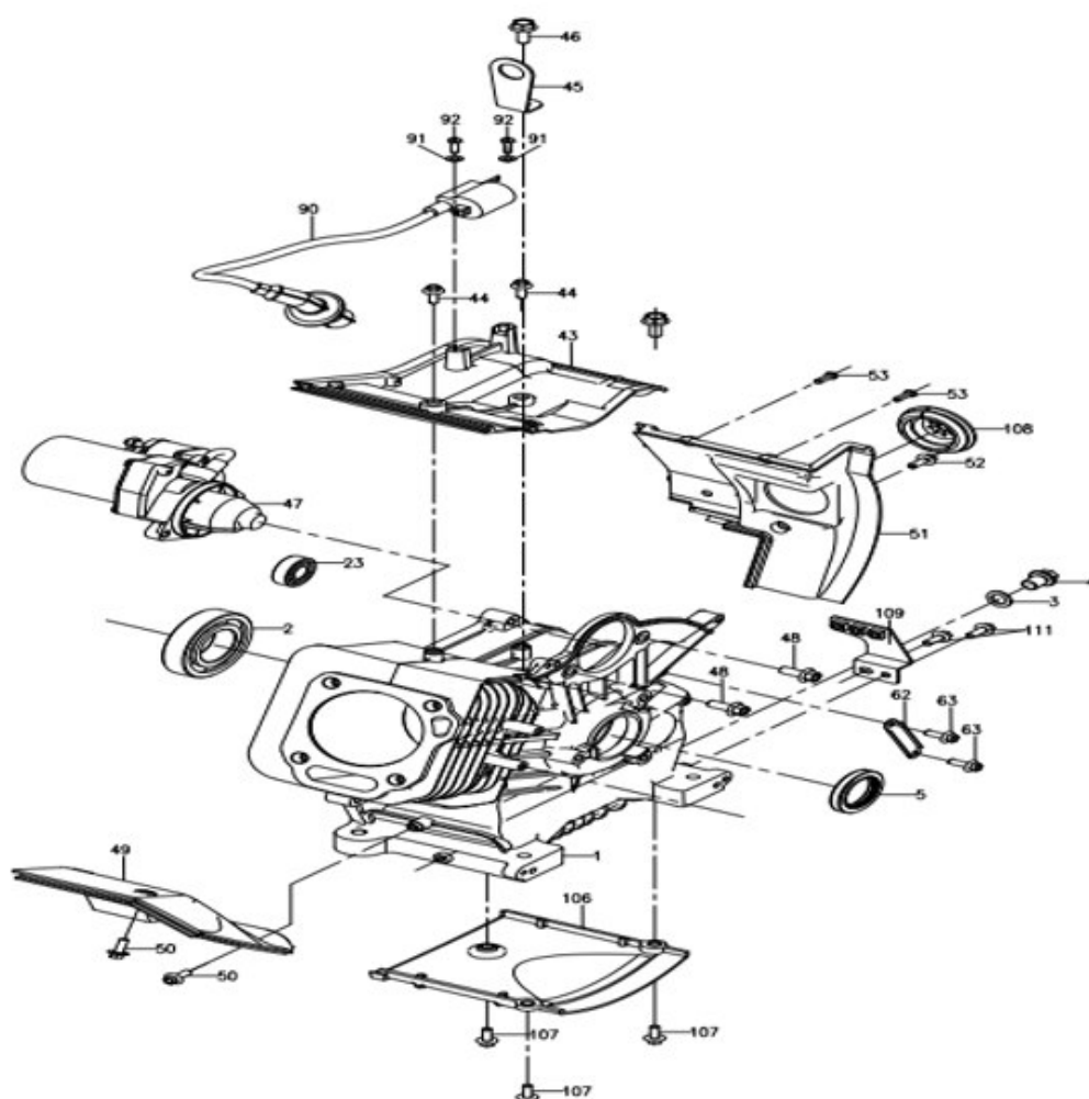
Abb. 10-31: Ersatzteilzeichnung 3
