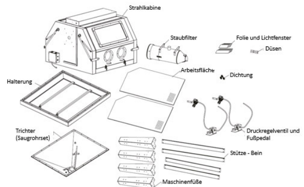
Abb. 4: Montageteile
