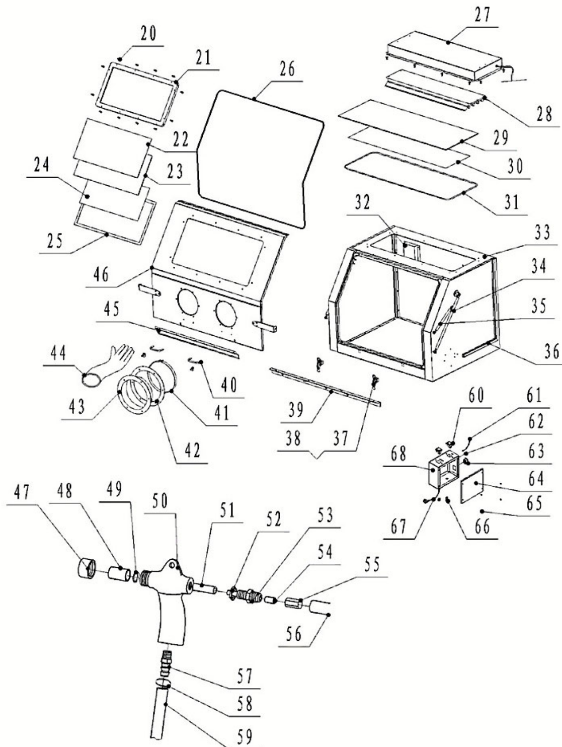
Abb. 9: Ersatzteilzeichnung 2 SSK 4
