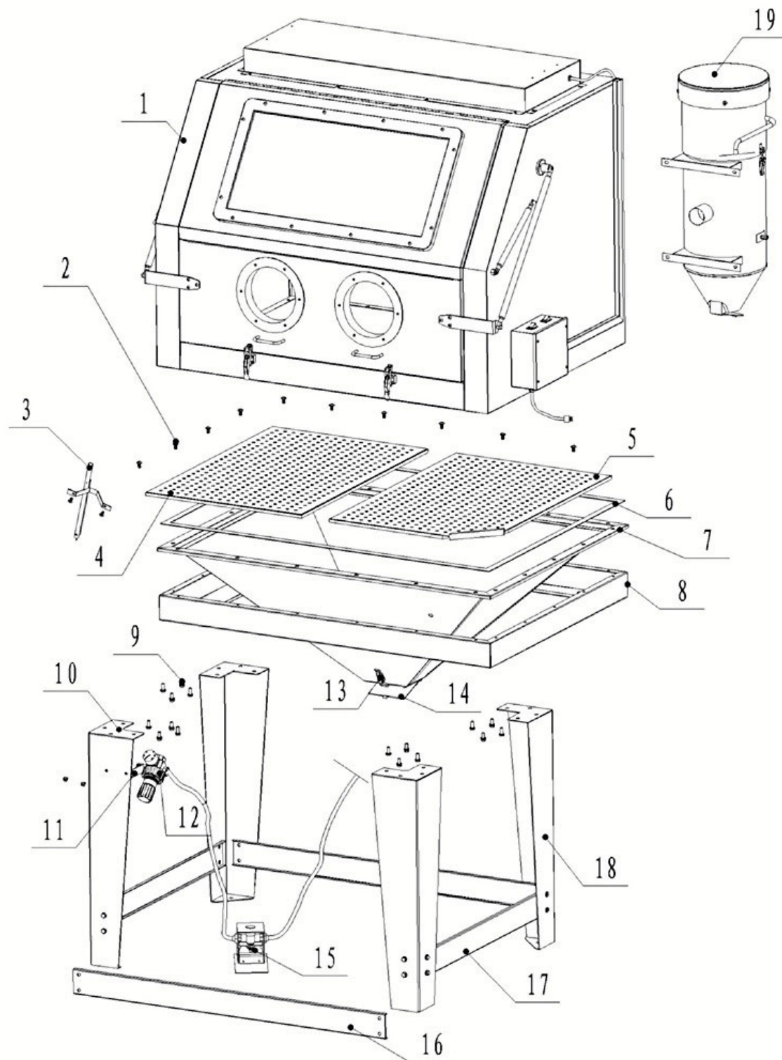
Abb. 8: Ersatzteilzeichnung 1 SSK 4
