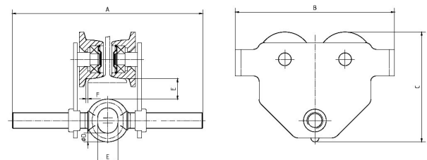
Abb. 2: Maße
