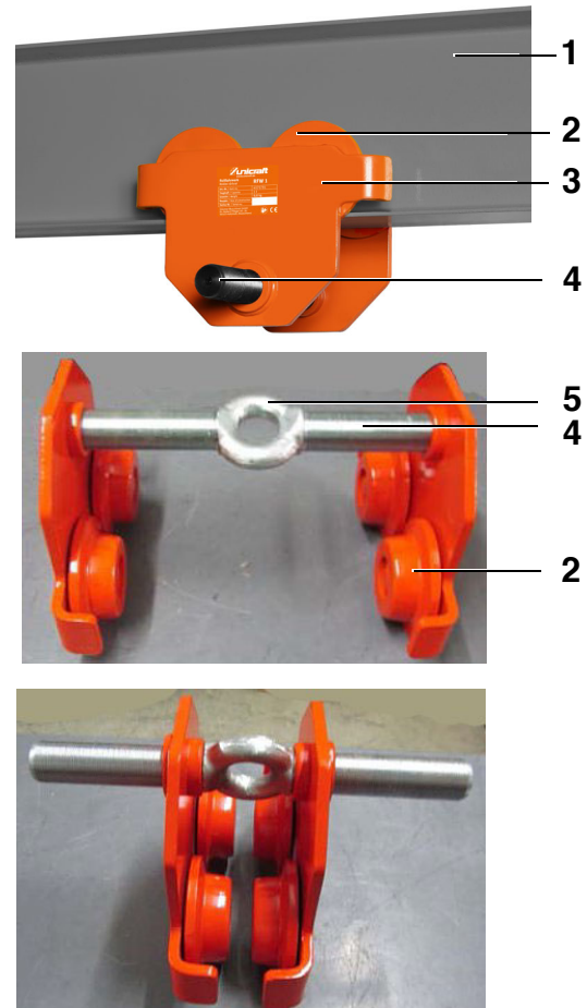
Abb. 4: Bauteile
