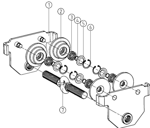
Abb. 8: Ersatzteilzeichnung RFW
