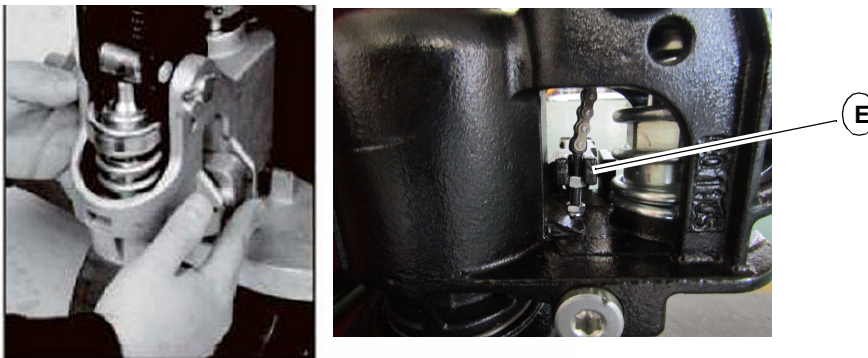
Abb.5-4: Kette befestigen
