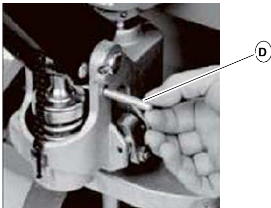
Abb. 5-2: Sicherungstift entfernen
