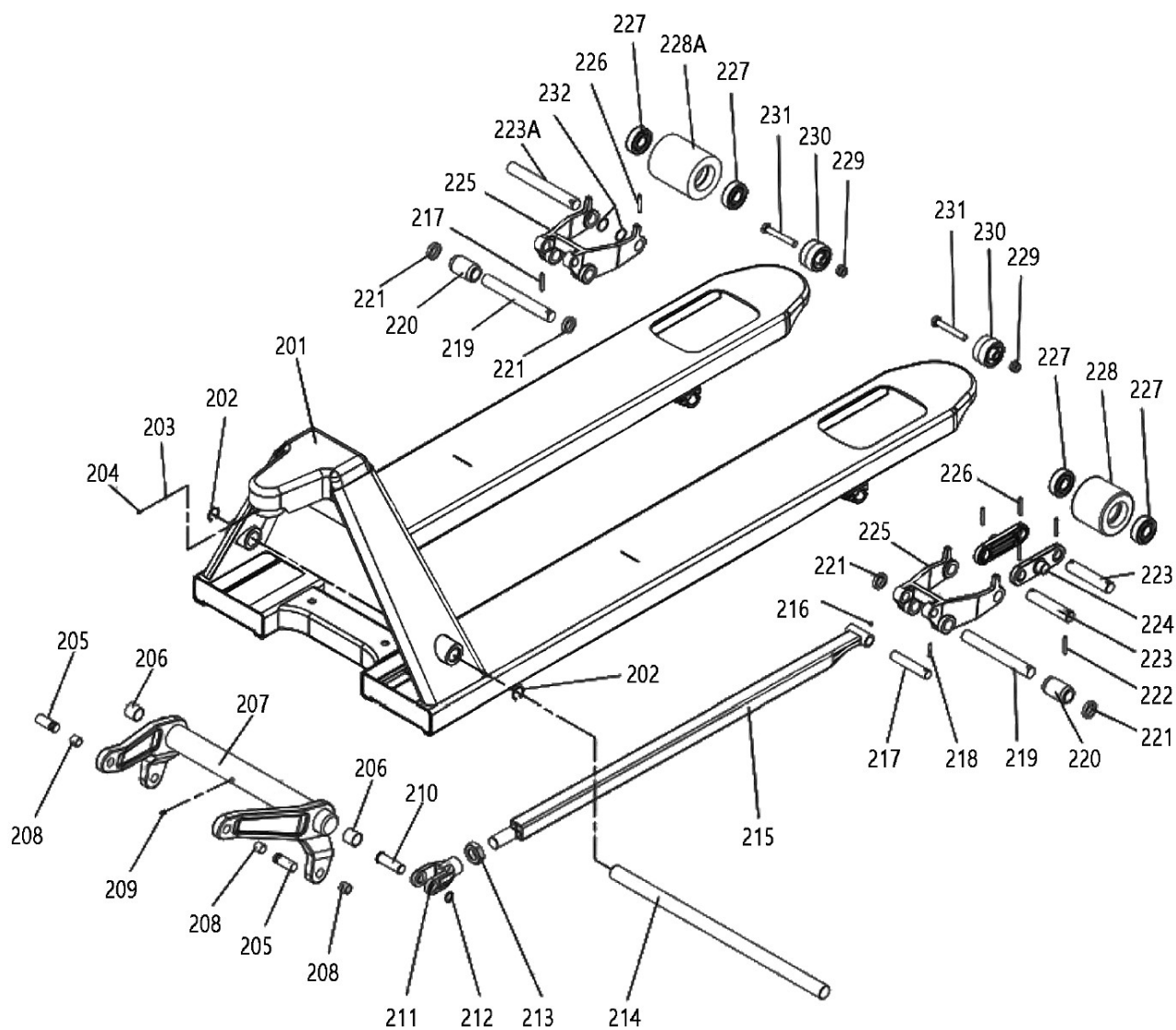
Abb. 10-1: Ersatzteilzeichnung 1
