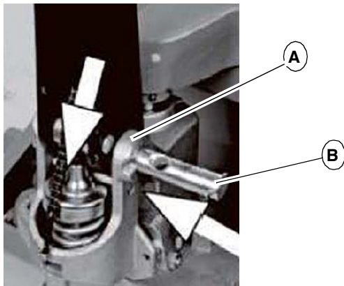
Abb. 5-1: Montage der Deichsel
