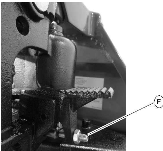
Abb. 6-1: Einstellung Hebelfunktionen
