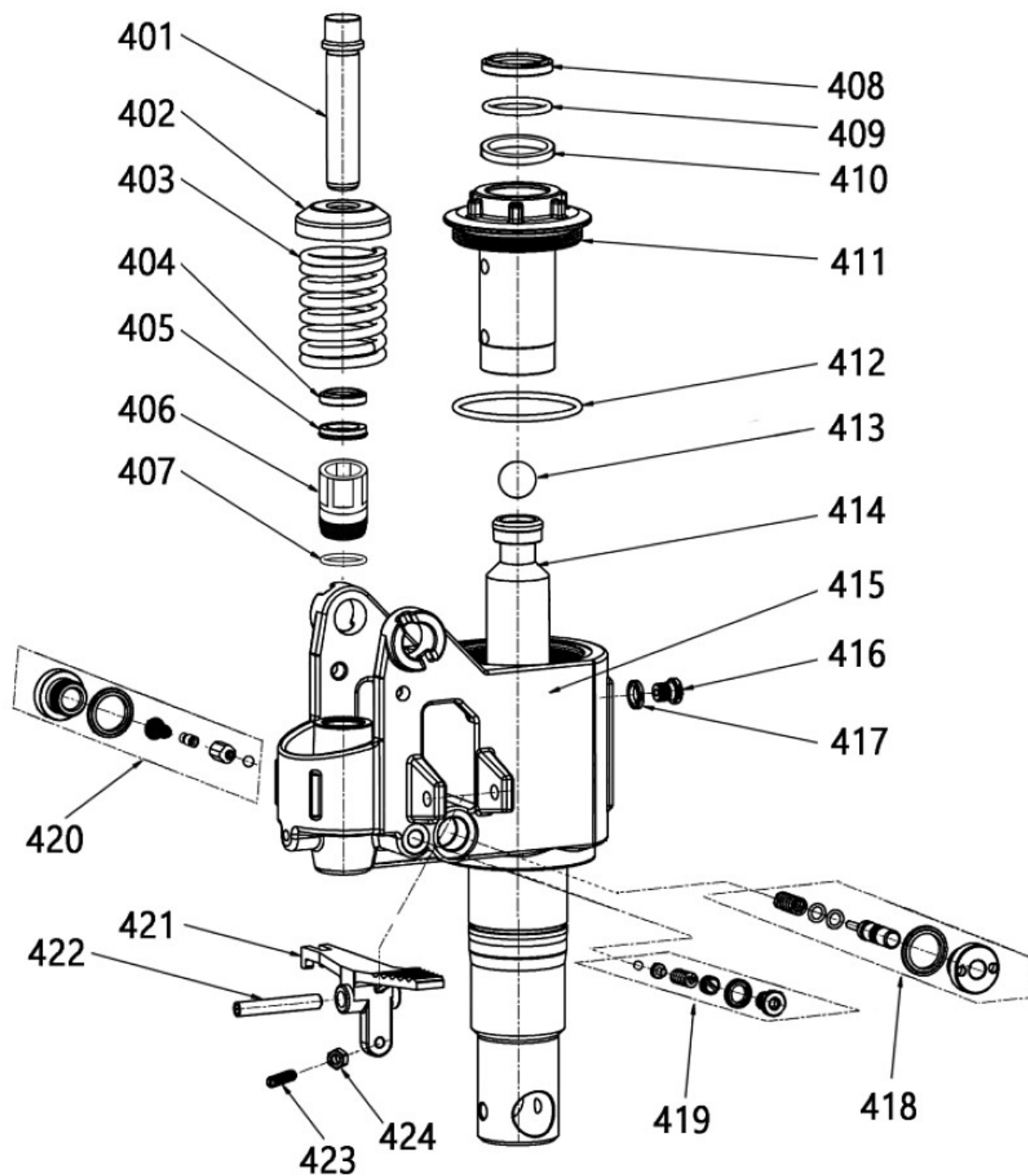
Abb.10-4: Ersatzteilzeichnung 4
