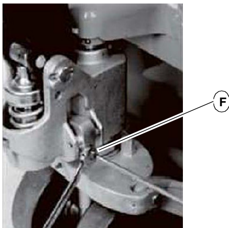
Abb.5-5: Hubgabel einstellen
