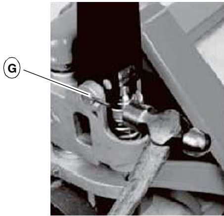
Abb. 5-6: Hubwagen entlüften
