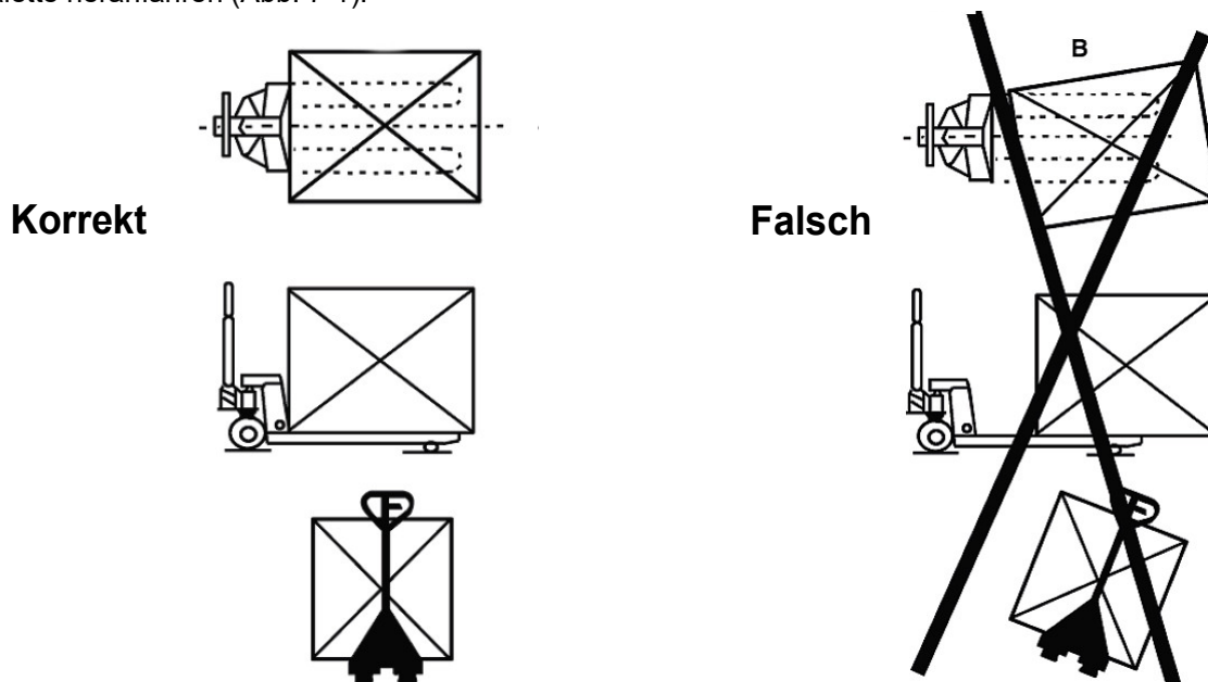
Abb.7-1: Last anheben und Transportieren
