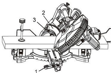
KGZ 3050
