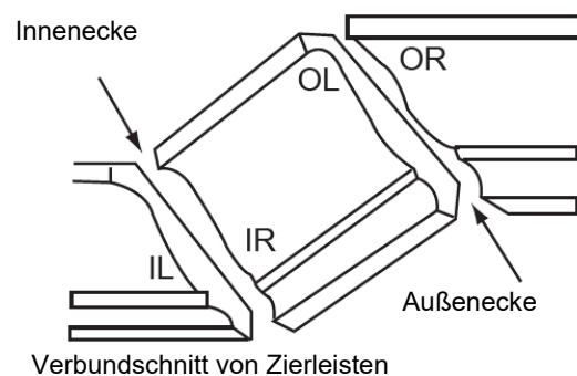
Abb. 43: Verbundzierleisten schneiden
