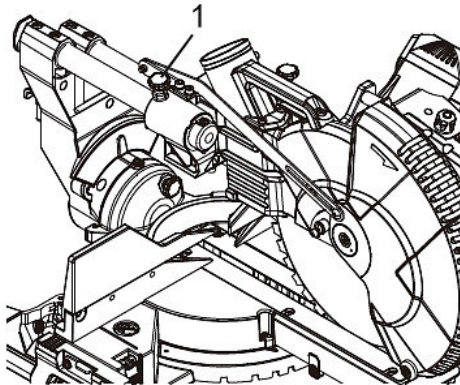
Abb. 36: Schiebeschlittensystem
