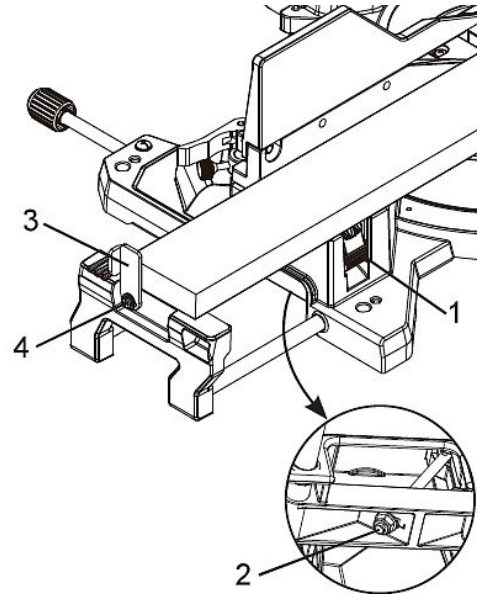
Abb. 26: Einstellung des Erweiterungsflügels
