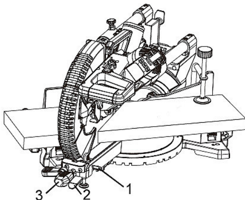
Abb. 38: Gehrungsschnitt
