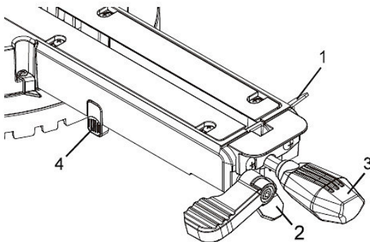
Abb. 37: Schnellnockenverriegelungshebel
