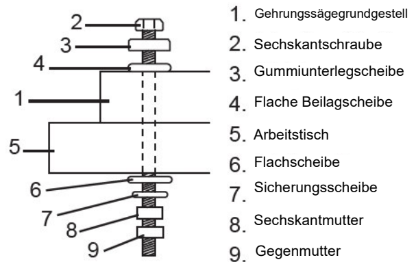
Abb. 15: Befestigung der Säge
