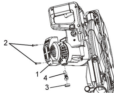
Abb. 49: Inspektion der Kohlebürsten
