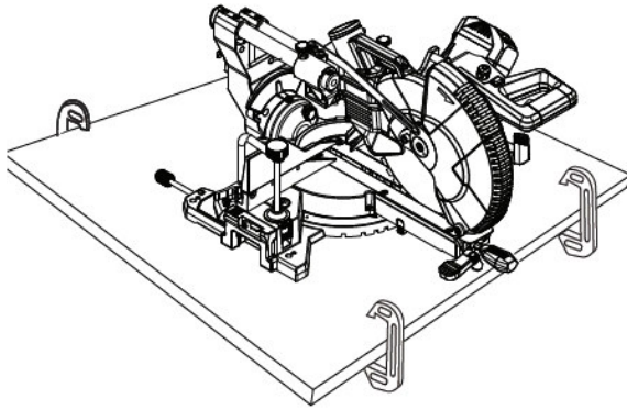
Abb. 16: Befestigung der Säge
