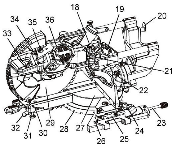
Abb. 5: Kapp- und Gehrungssäge KGZ 3050 Vario
