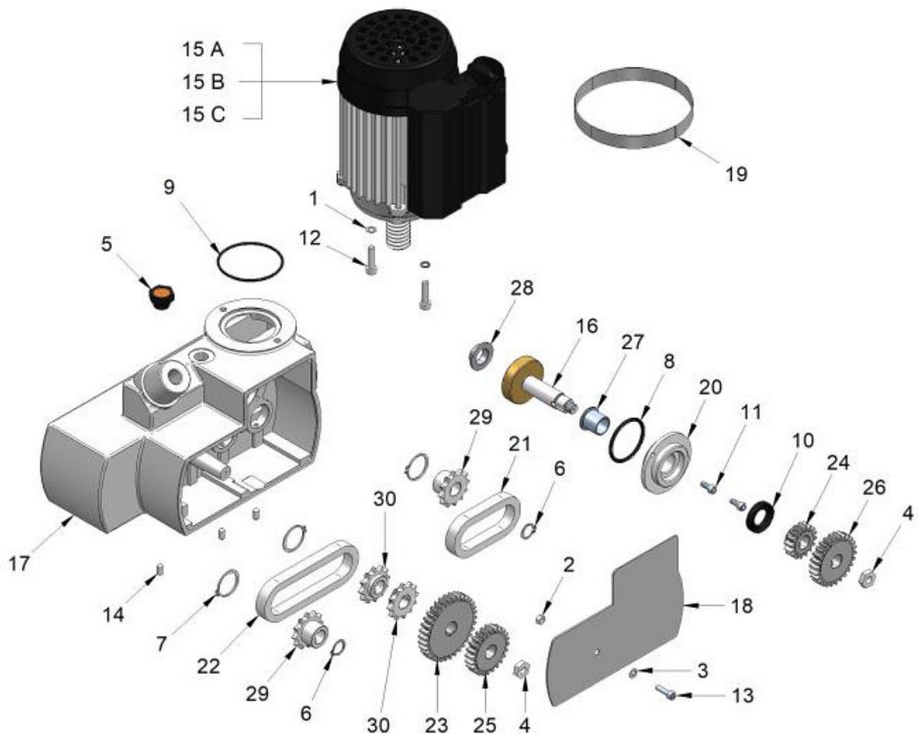
Abb. 13-1: Ersatzteilzeichnung 1
