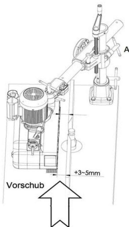
Abb.9-1: Senkrechte Nutzung des Vorschubapparats
