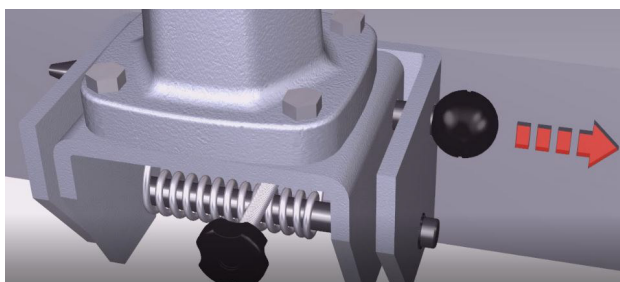
Abb. 6-9: Wegklappvorrichtung schwenken
