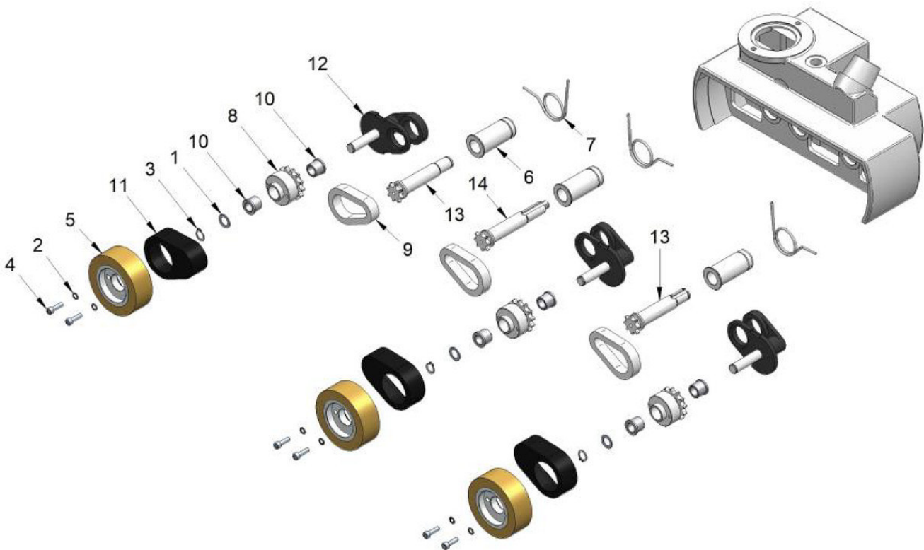
Abb.13-2: Ersatzteilzeichnung 2
