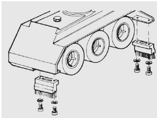
Abb.6-4: Montage der Schutzbürsten
