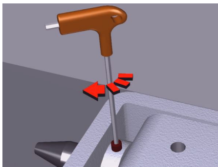
Abb. 6-7: Wegklappvorrichtung fixieren
