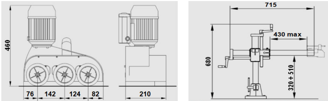
Abb.4-5: Abmessungen VSA 2033
