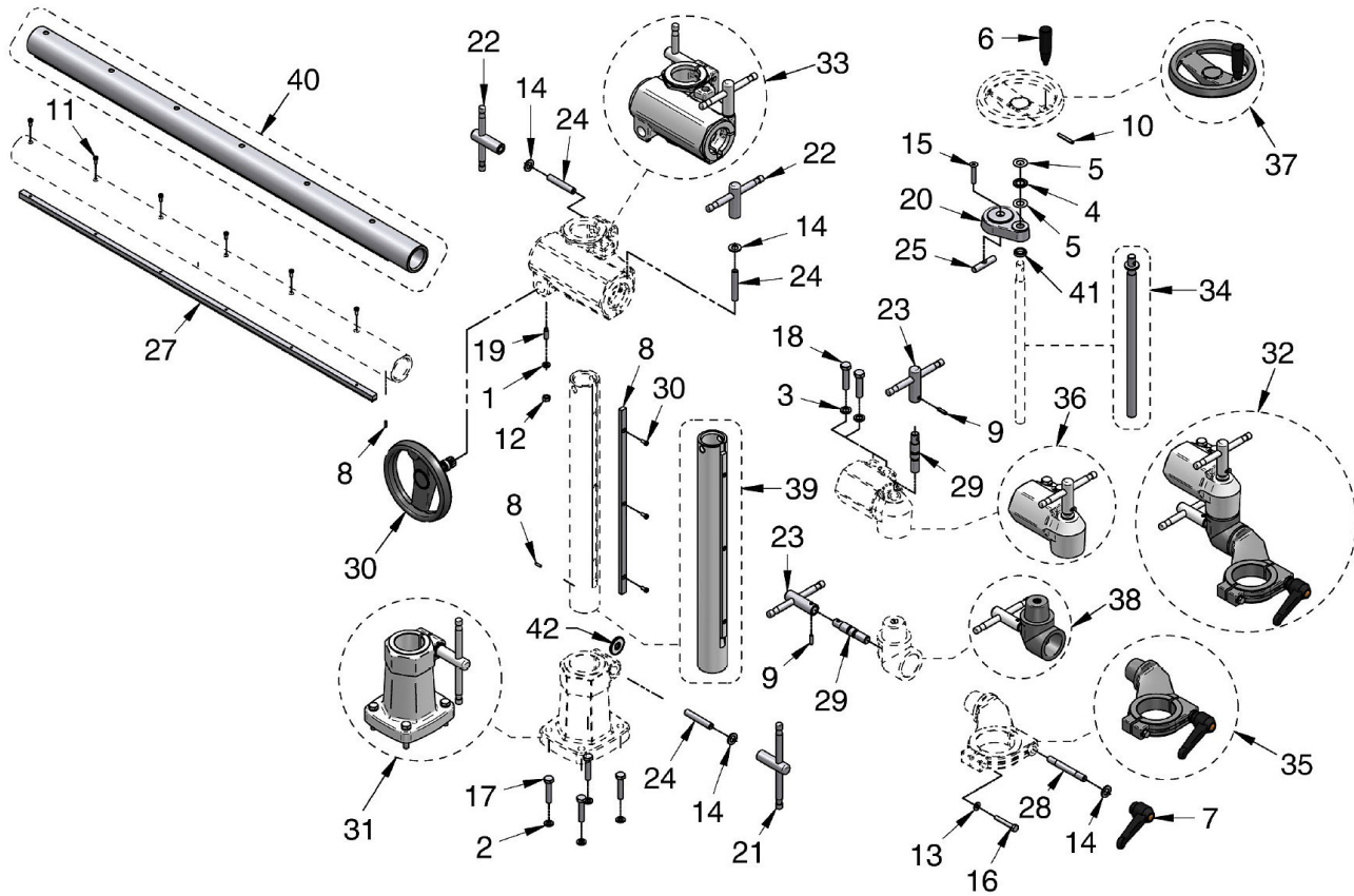
Abb. 13-18: Ersatzteilzeichnung Stativ 1050
