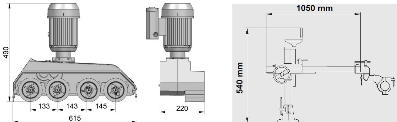
Abb. 4-11: Abmessungen VSA 4V DC
