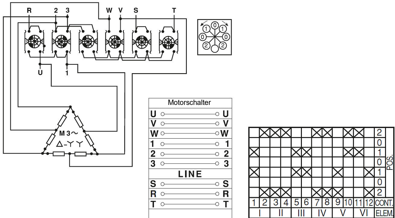
Abb. 13-22: Elektroschaltplan 2 VSA 2038 L, VSA 2038 L PLUS, VSA 2048 L, VSA 2048 L PLUS
