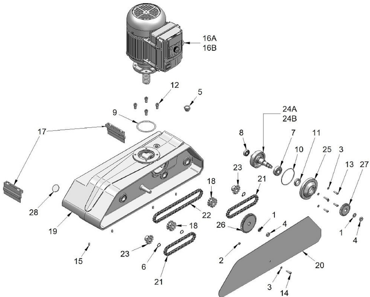
Abb. 13-11: Ersatzteilzeichnung 1
