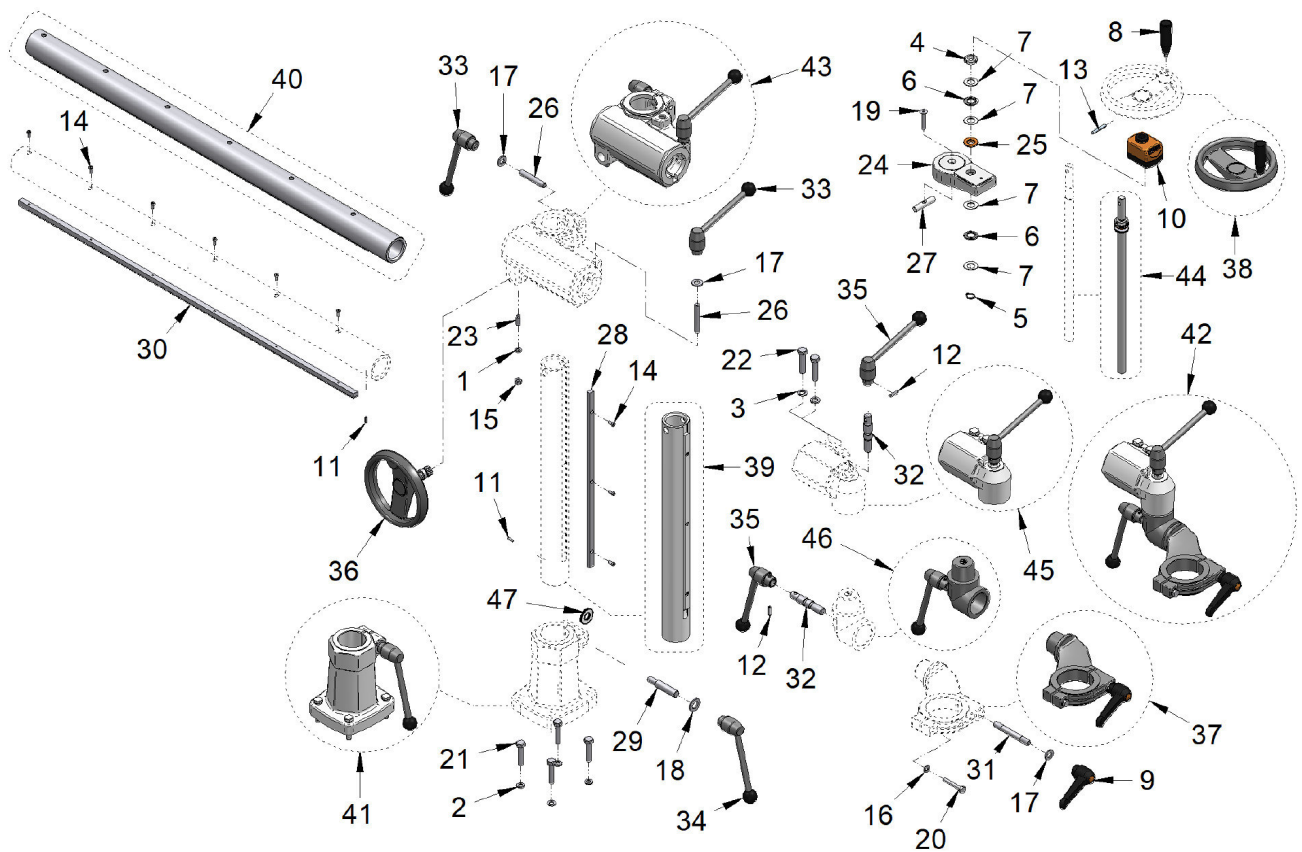
Abb. 13-19: Ersatzteilzeichnung Stativ 1050 PLUS
