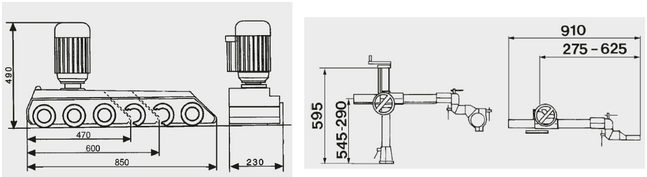
Abb. 4-7: Abmessungen VSA 2038L Plus und VSA 2048L Plus
