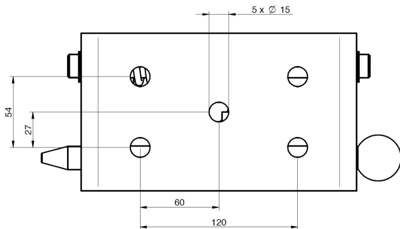
Abb. 6-6: Bohrungsabstand Wegklappvorrichtung an die Maschine
