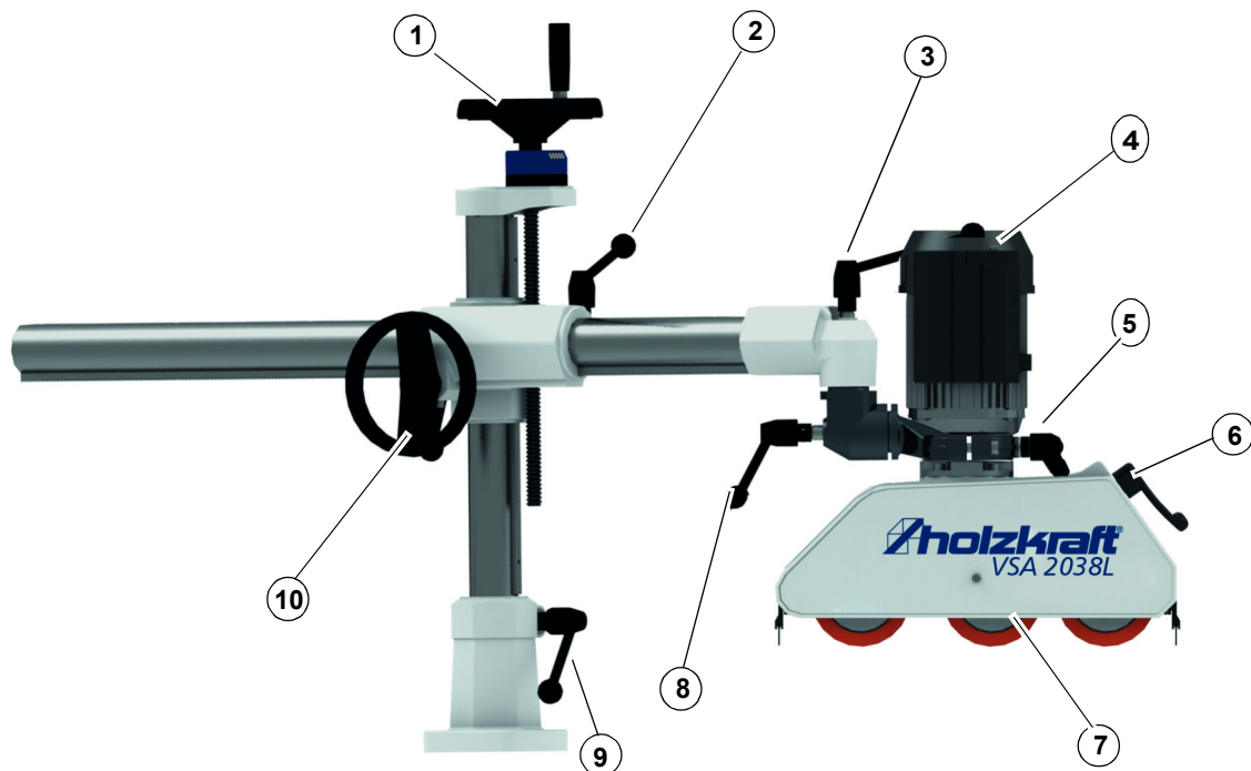
Abb.4-6: VSA 2038L mit Plus Stativ
