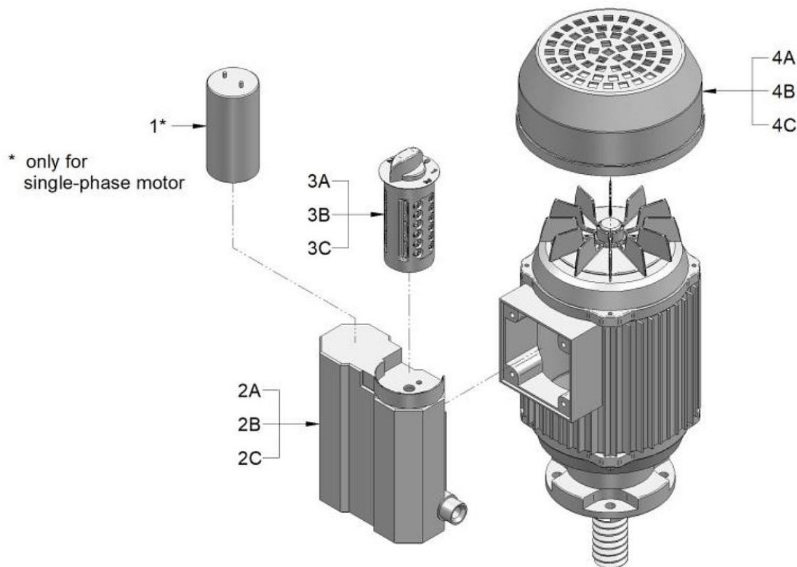
Abb. 13-3: Ersatzteilzeichnung 3
