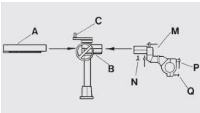
Abb.6-1: Montage des Stativs
