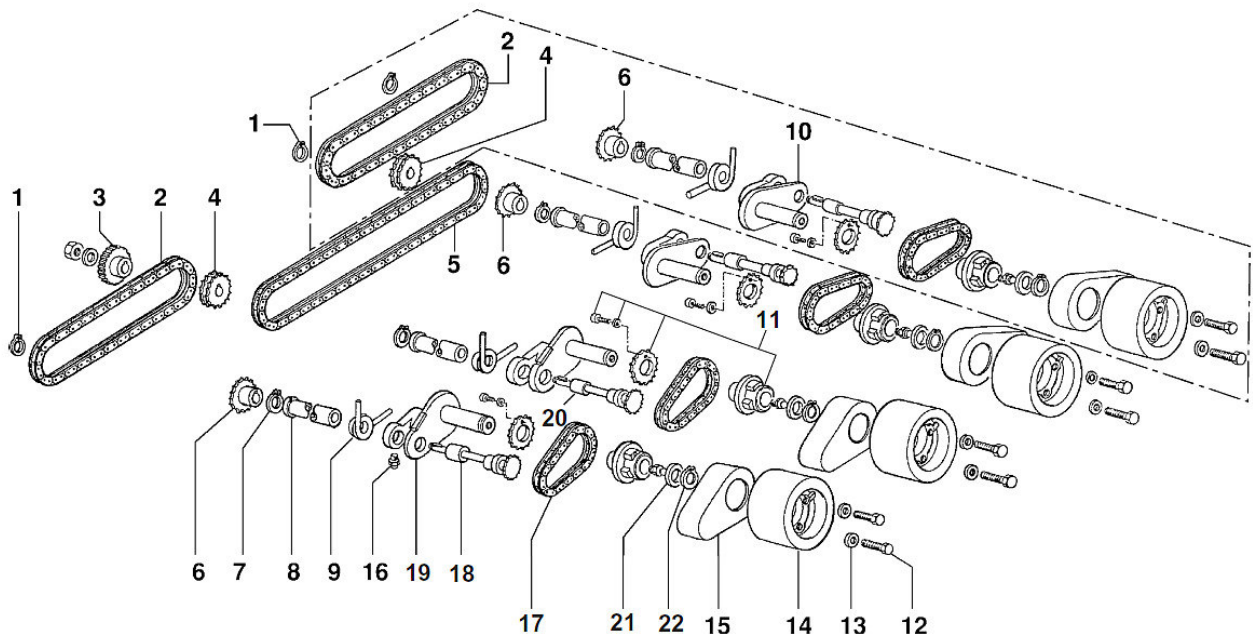
Abb. 13-6: Ersatzteilzeichnung 2
