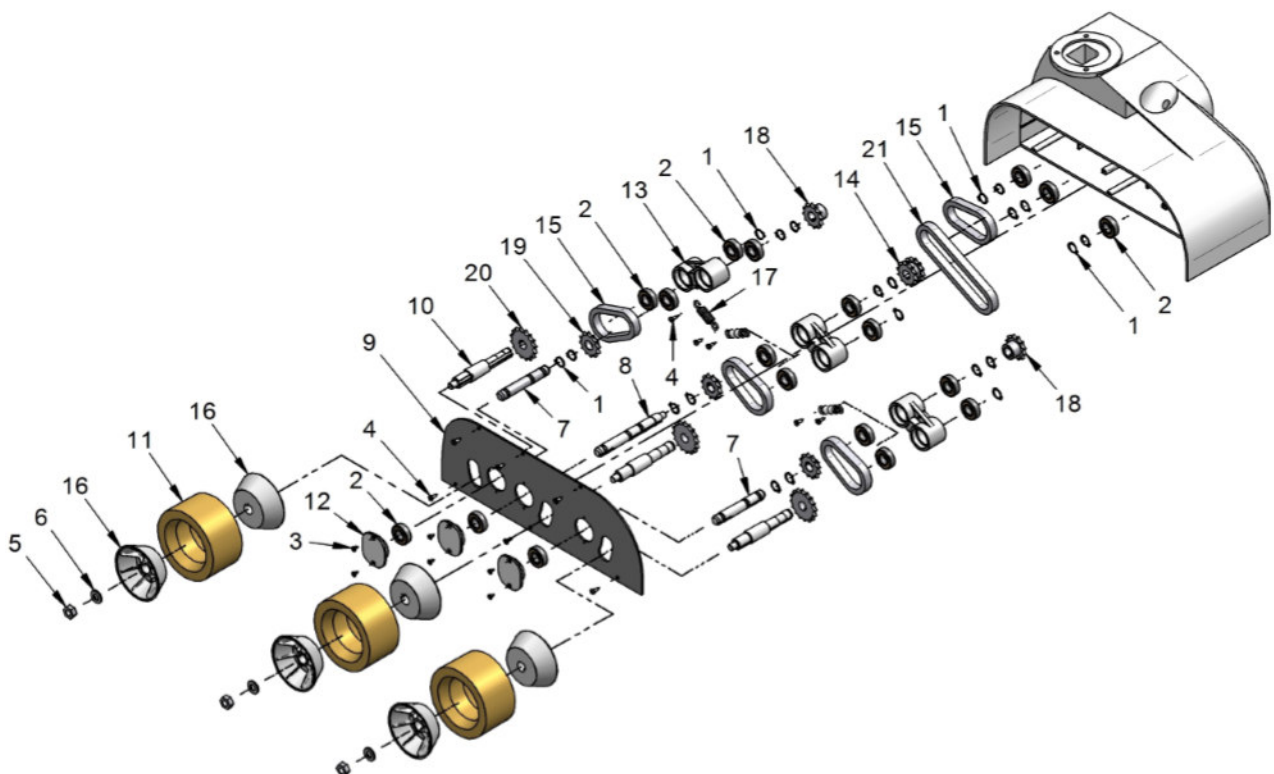
Abb. 13-15: Ersatzteilzeichnung 2
