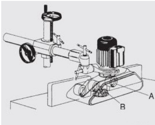
Abb. 10-2: Anbringen an einer Tischfräsmaschine
