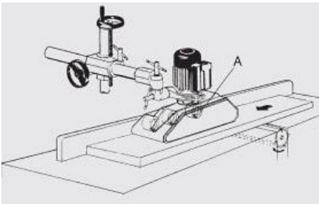
Abb. 10-3: Anbringen an einer Abrichthobelmaschinen
