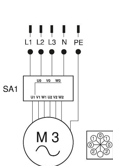
Abb. 13-21: Elektroschaltplan 1 VSA 2038 L, VSA 2038 L PLUS, VSA 2048 L, VSA 2048 L PLUS
