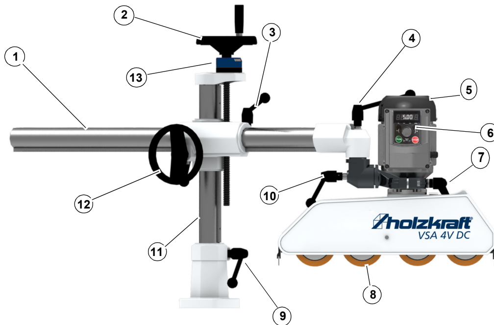
Abb.4-10: VSA 4V DC
