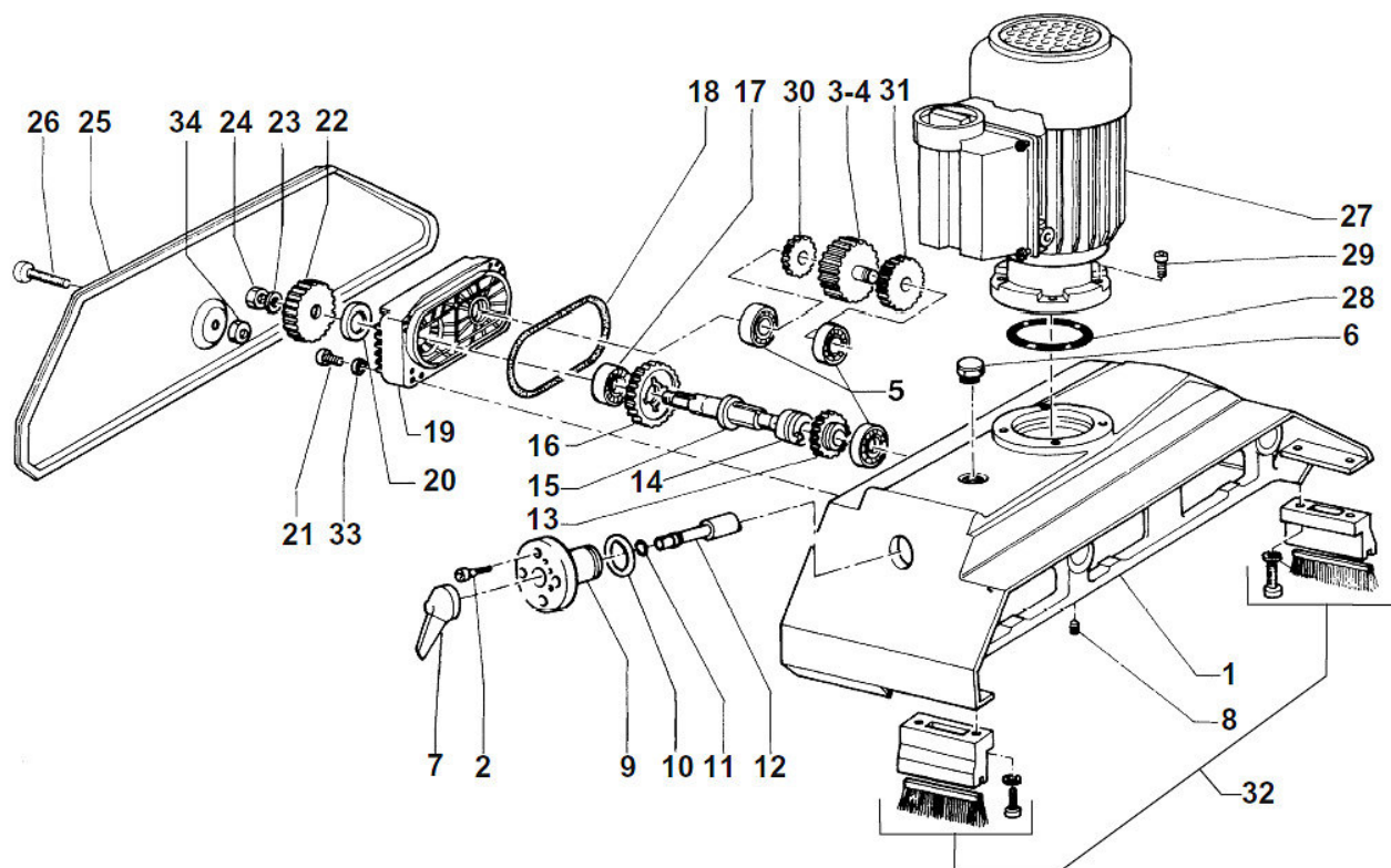
Abb.13-5: Ersatzteilzeichnung 1
