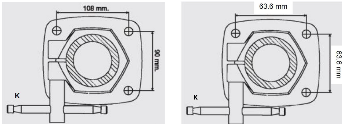
Abb. 6-2: Montage Stativ an die Maschine (VSA 2033, VSA 2038, VSA 2048 links; VSA 2032 rechts)
