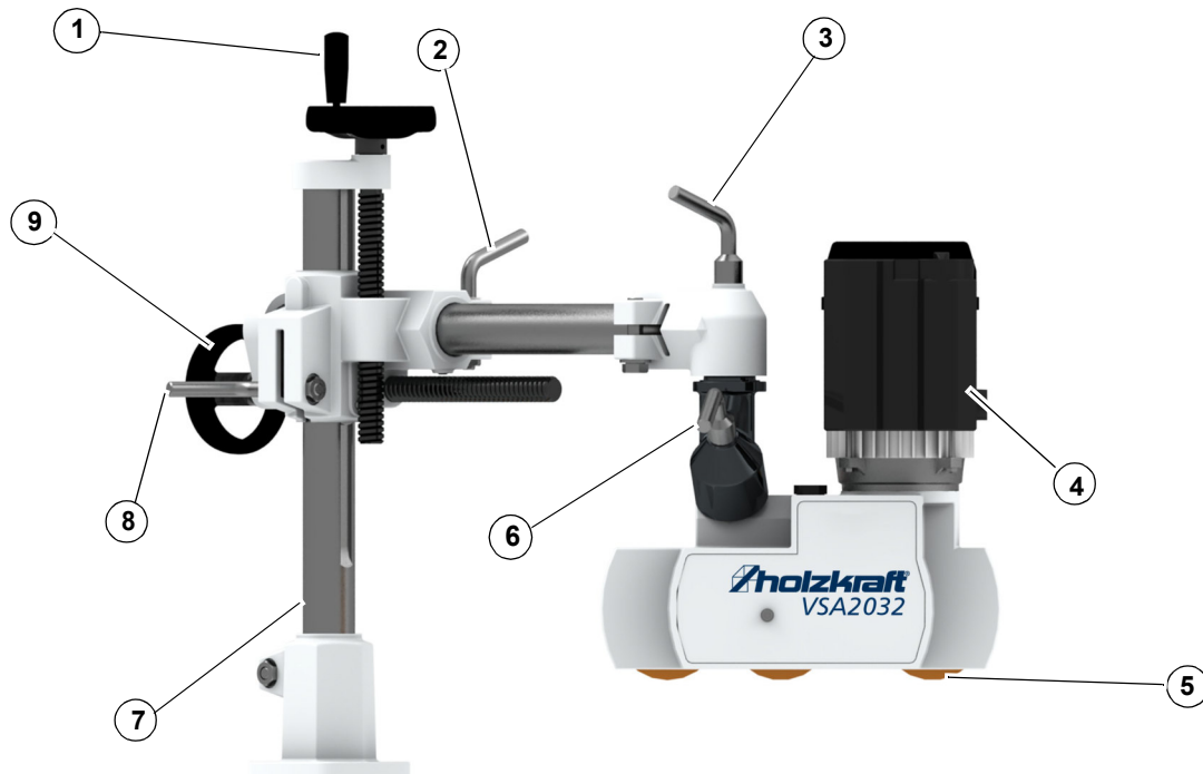
Abb.4-1: VSA 2032
