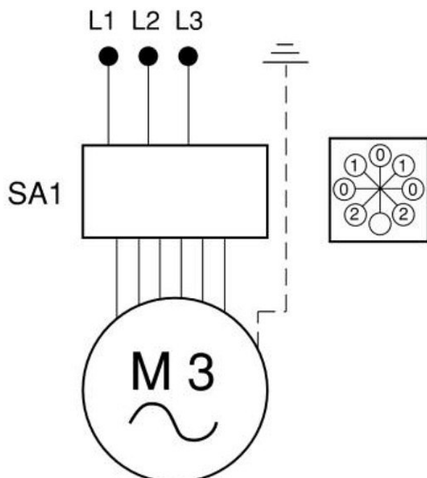
Abb. 13-20: Elektroschaltplan VSA 2032, VSA 4 V, VSA 4V DC
