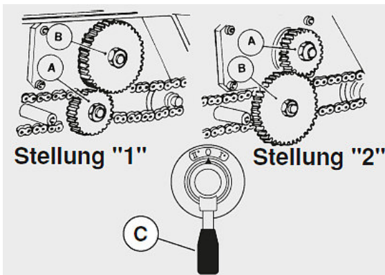
Abb. 7-5: Einstellung Geschwindigkeit VSA 2038 L bis VSA 2048 L PLUS
