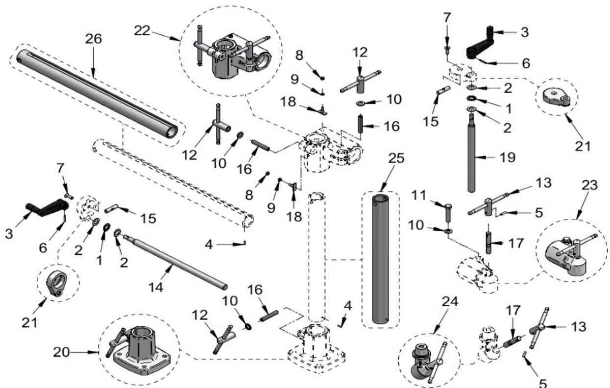
Abb. 13-17: Ersatzteilzeichnung 4
