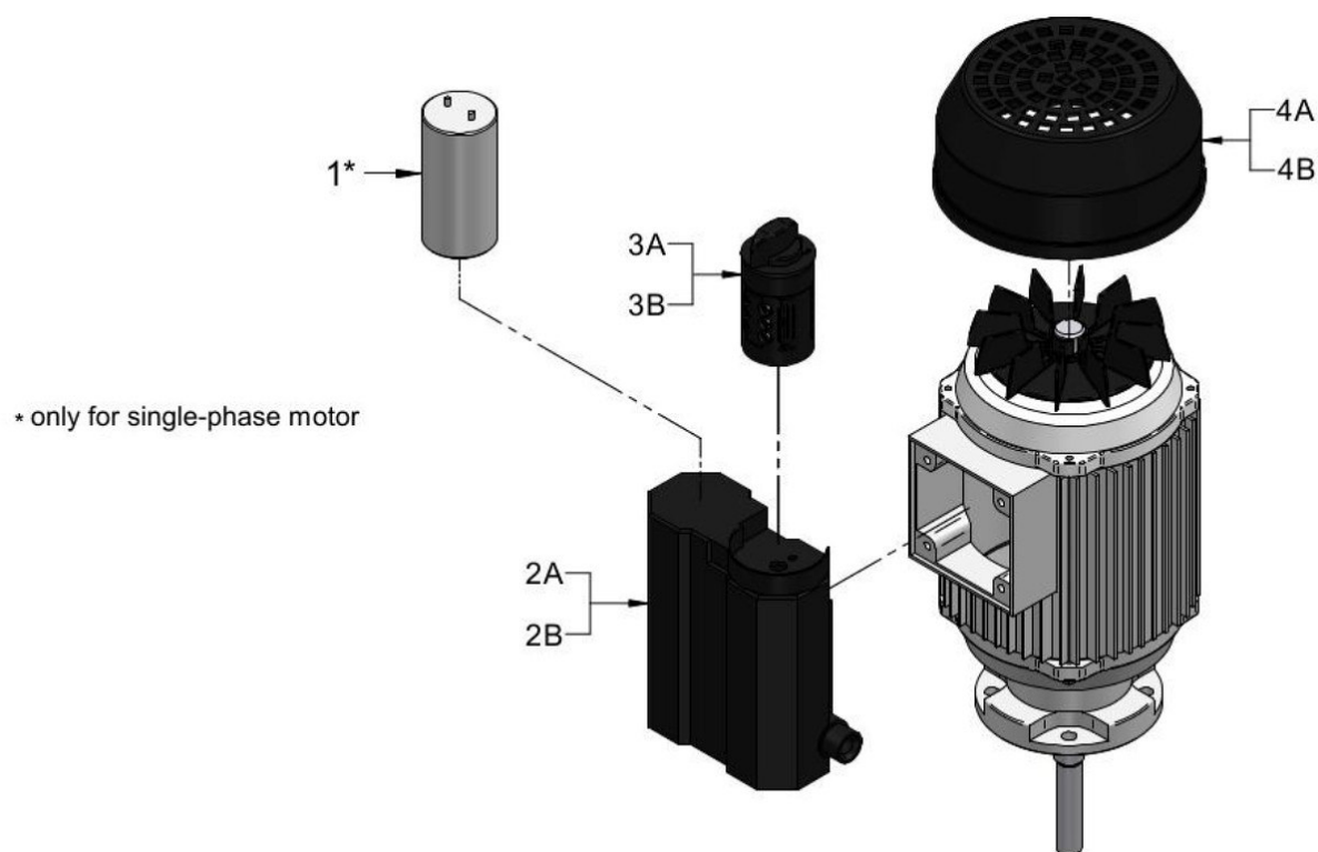
Abb. 13-10: Ersatzteilzeichnung 3
