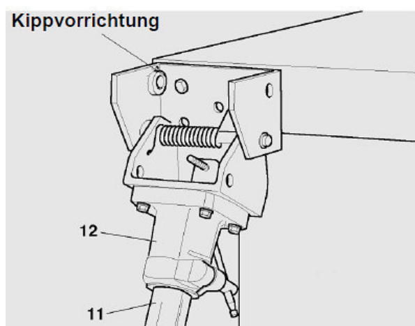
Abb.6-5: Montage Wegklappvorrichtung (Zubehör)
