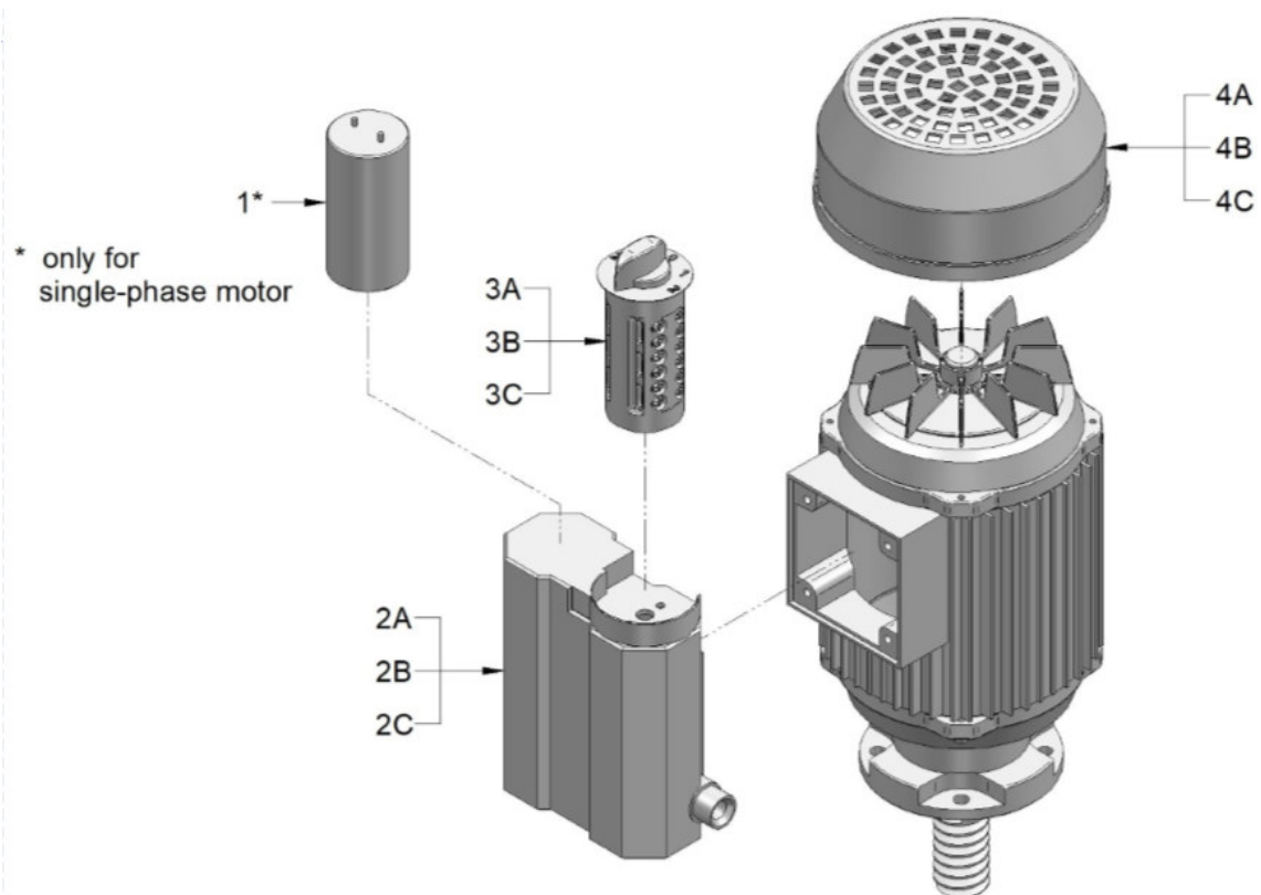
Abb. 13-16: Ersatzteilzeichnung 3
