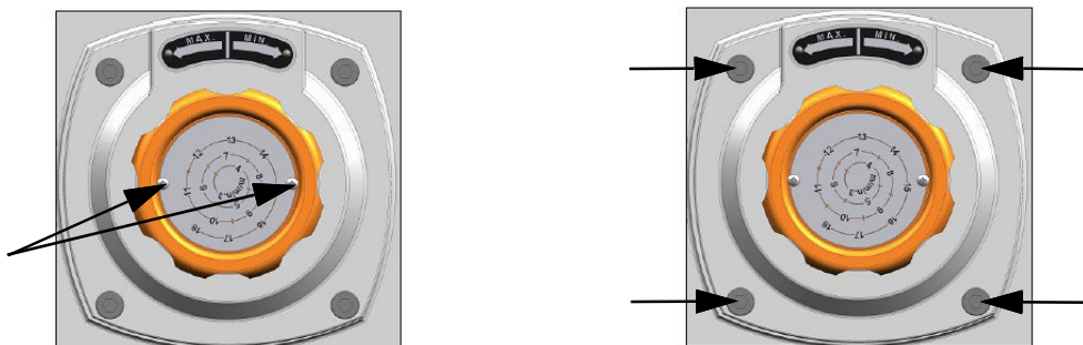
Abb. 11-2: Abdeckung Drehknopf öffnen (links), Gehäuse demontieren (rechts)
