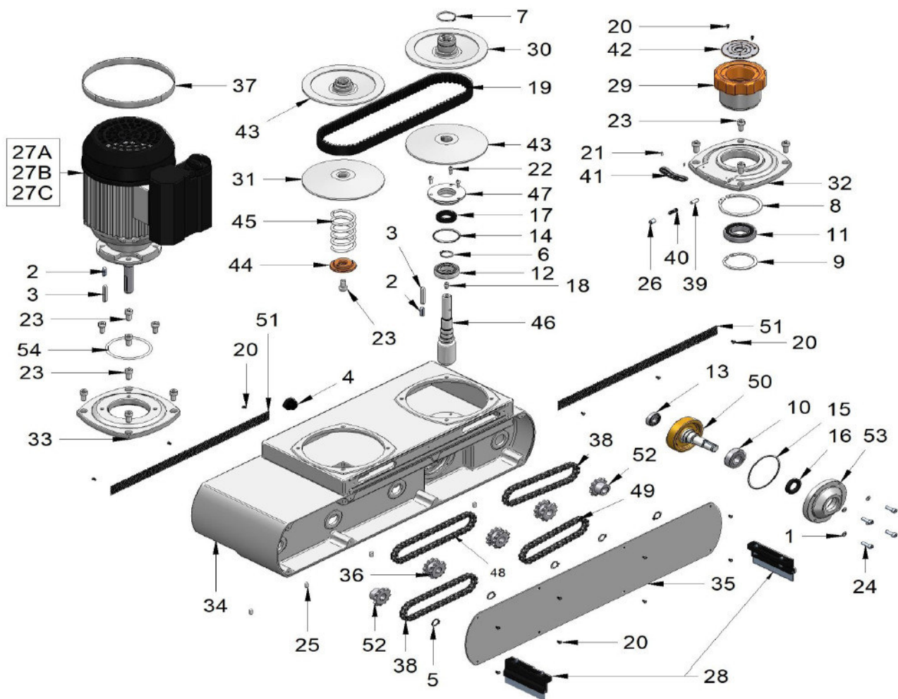
Abb.13-8: Ersatzteilzeichnung 1
