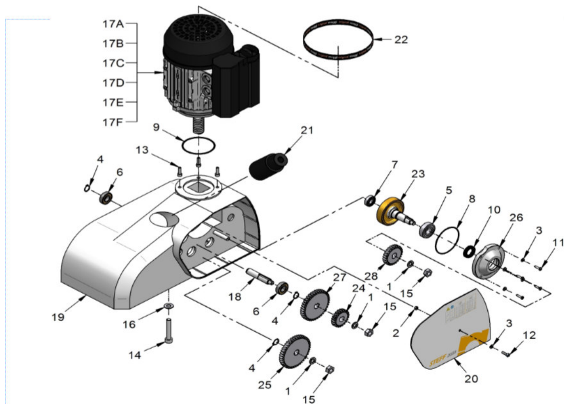
Abb. 13-14: Ersatzteilzeichnung 1
