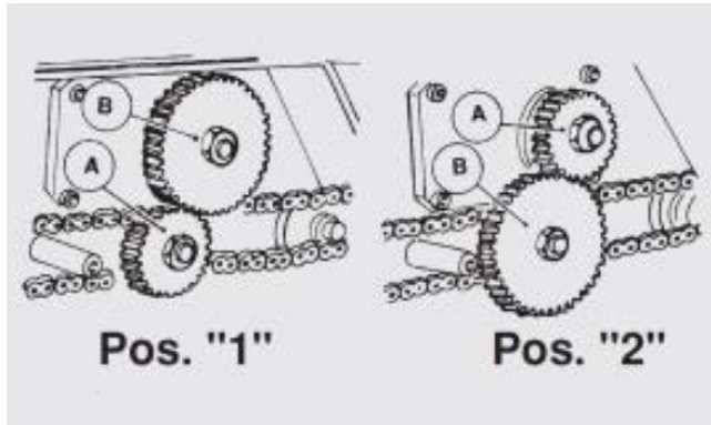
Abb. 7-4: Einstellung Geschwindigkeit VSA 2032
