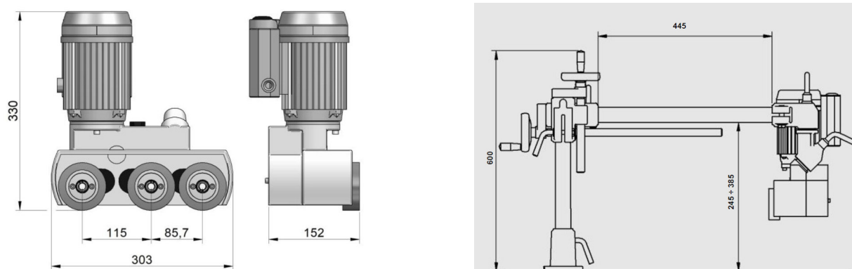
Abb.4-2: Abmessungen VSA 2032
