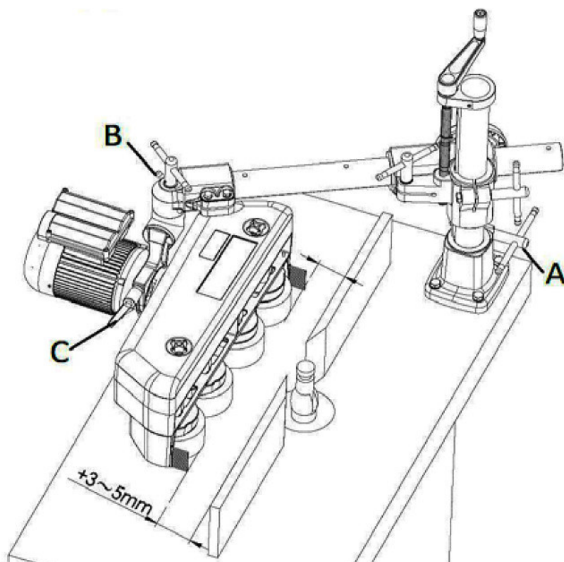
Abb. 9-2: Waagrechte Nutzung des Vorschubapparats
