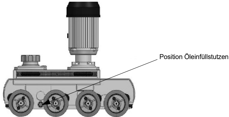
Abb. 11-3: Position Öleinfüllstutzen
