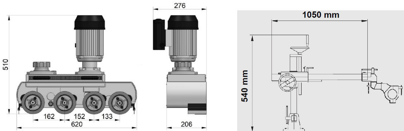
Abb.4-9: Abmessungen VSA 4V
