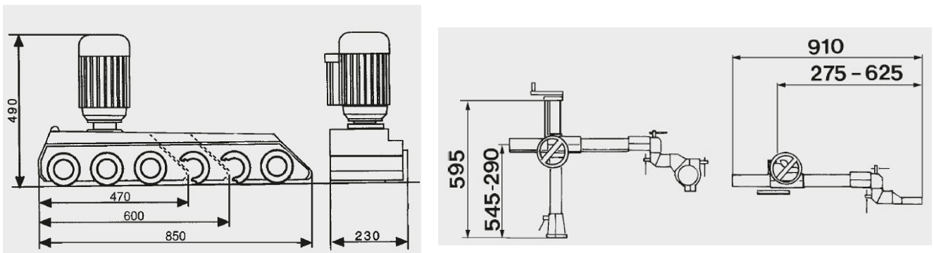
Abb. 4-4: Abmessungen VSA 2038 L und VSA 2048L
