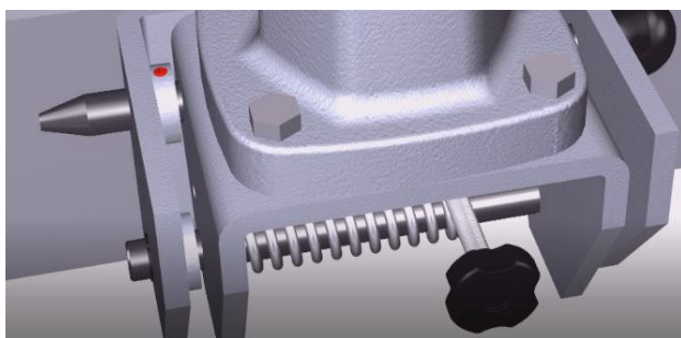
Abb. 6-8: Wegklappvorrichtung fixieren
