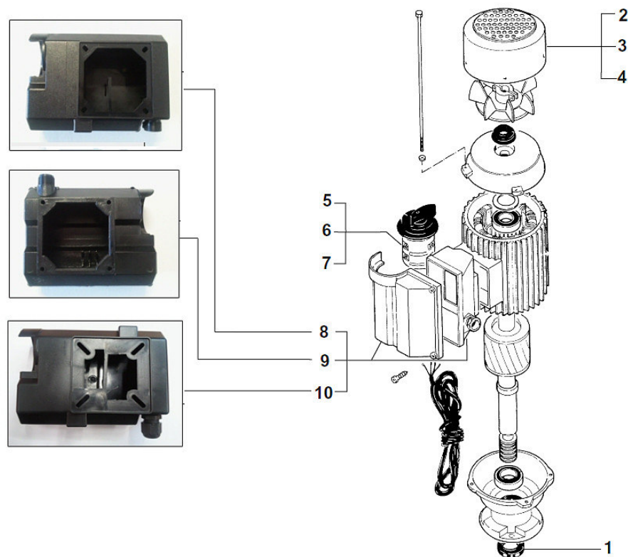
Abb. 13-7: Ersatzteilzeichnung 3
