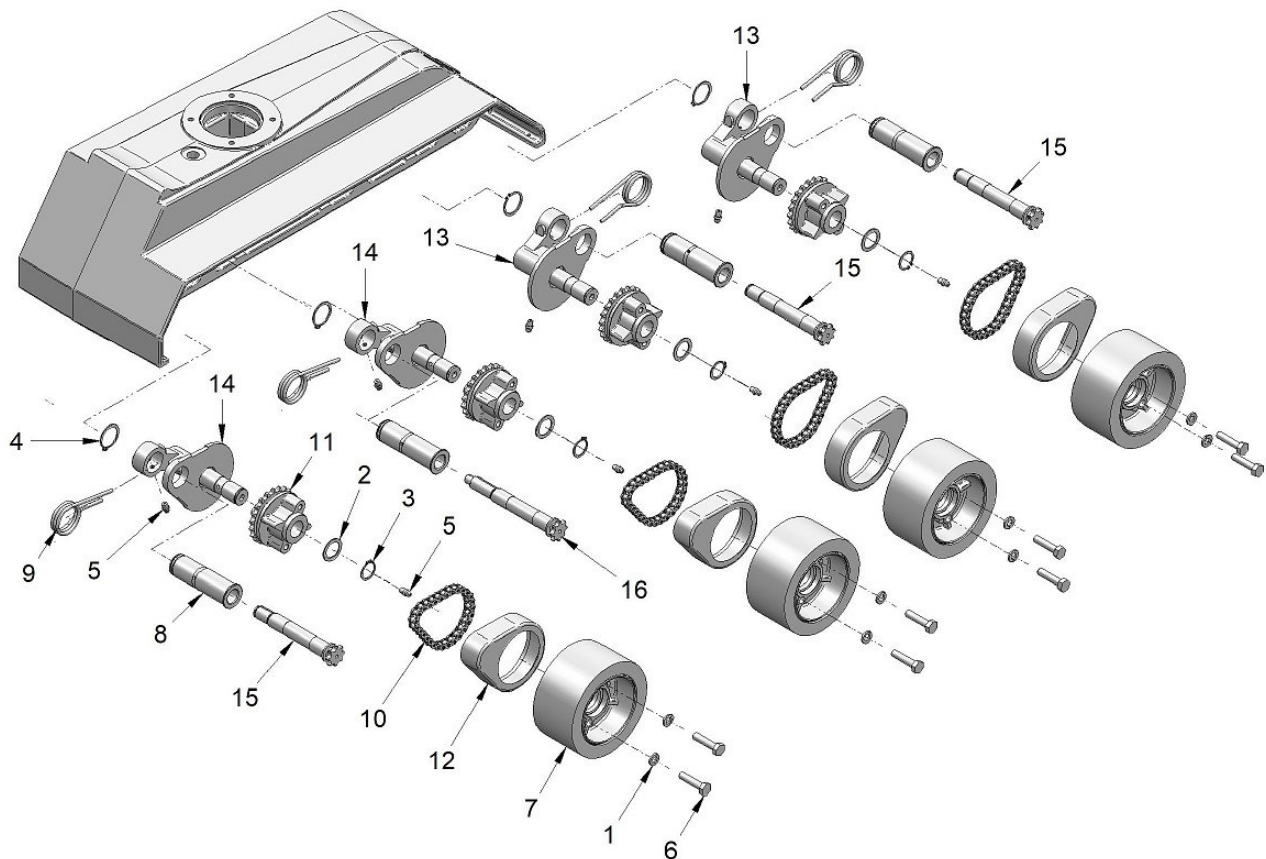
Abb. 13-12: Ersatzteilzeichnung 2
