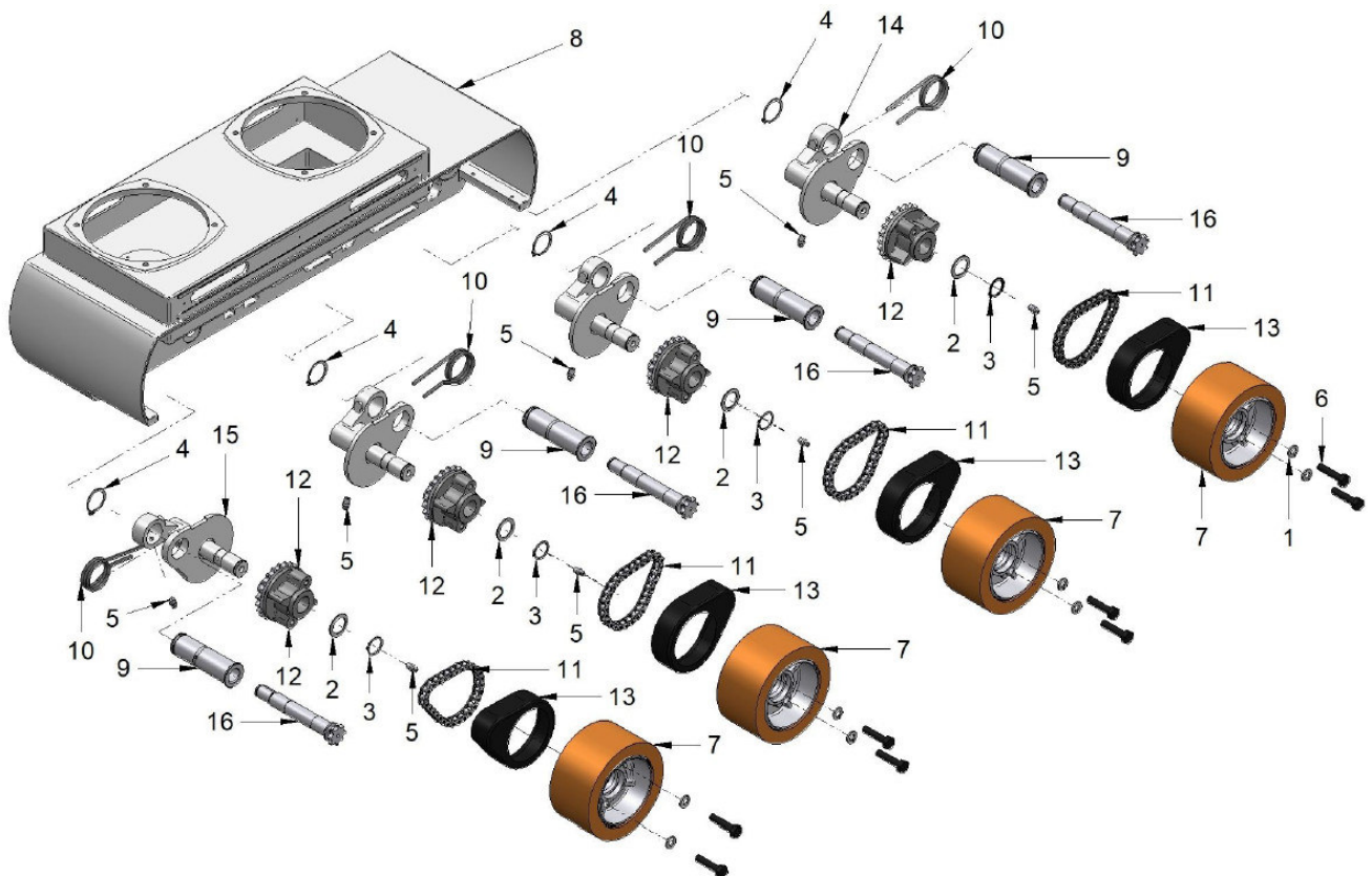
Abb. 13-9: Ersatzteilzeichnung 2
