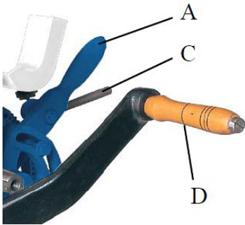
Abb. 11: Bedienhebel zur Bewegung der Hinterwalze
