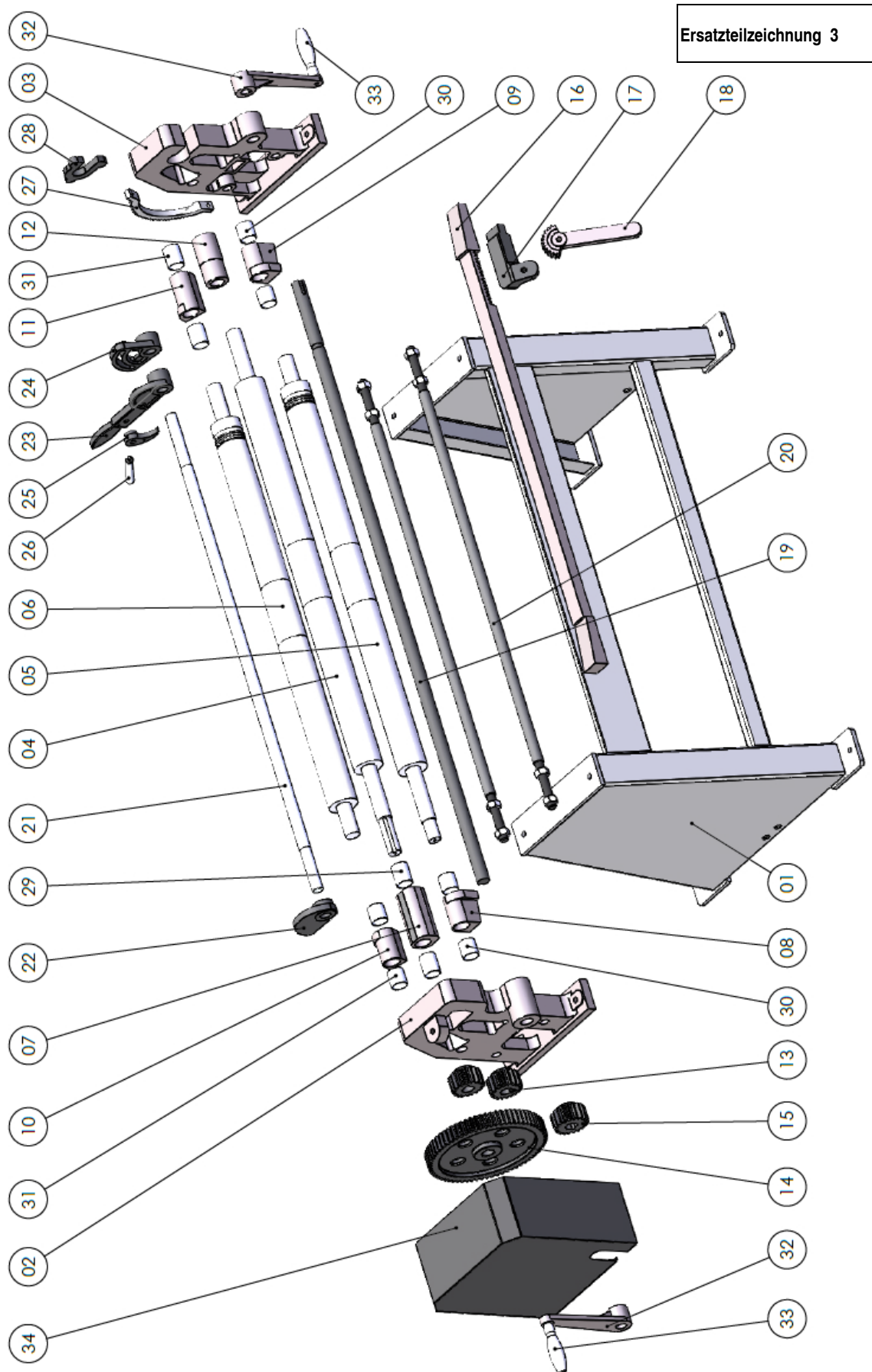
Abb. 19: Ersatzteilzeichnung 3: RBM 1050-22
