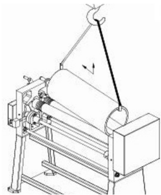
Abb. 15: Werkstück abstützen
