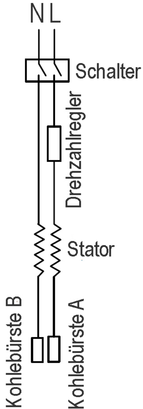
Abb. 4: Elektroschaltplan
